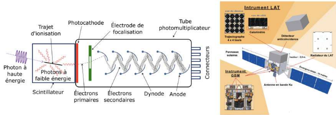
FIGURE 1.19 – Détecteurs du rayonnement de haute énergie. Schéma de principe d'un système scintillateur-photomultiplicateur (à gauche, Crédit : Wikimedia Commons ) et satellite Fermi, dont l'instrument GBM est composé d'une quinzaine de scintillateurs (à droite, Crédit : Wikimedia Commons ).
