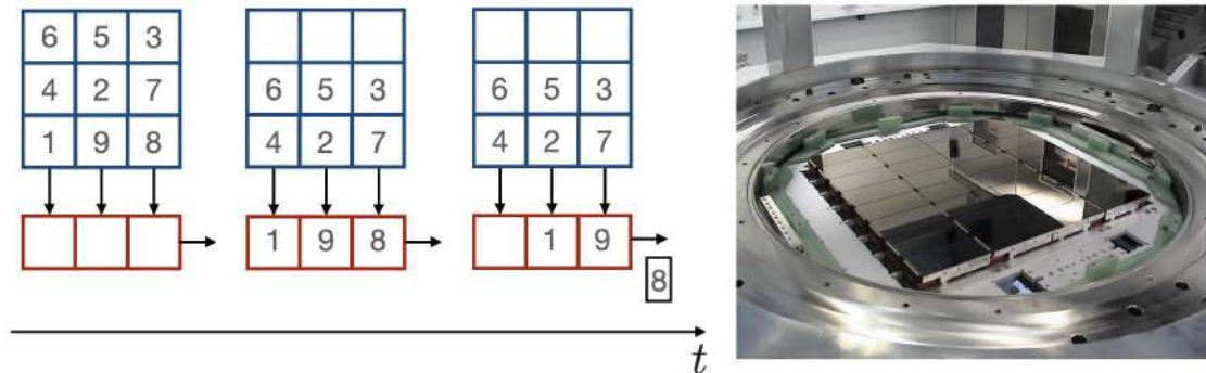
FIGURE 1.16 – Matrices CCD. Principe de lecture (à gauche) et matrice CCD (256 Megapixels) OmegaCAM du Very Large telescope (ESO/VLT).
