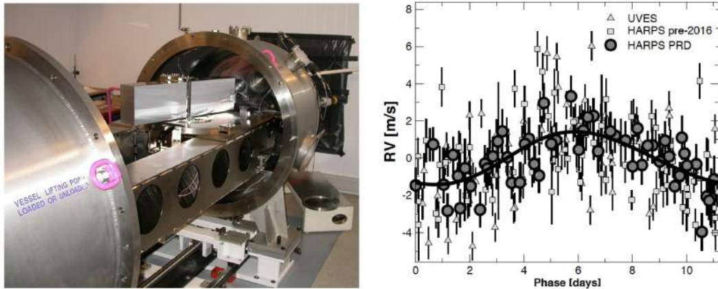
FIGURE 1.20 – Spectromètre HARPS. Photographie du dispositif montrant le réseau en réflexion (à gauche, Crédit : ESO/HARPS ) et mesures de la vitesse radiale de l'étoile Proxima Centauri avec (notamment) HARPS. Les données (représentées par les cercles, carrés et triangles) ont été prises au cours de 16 ans d'observations, et compilées pour faire ressortir, par ajustement (courbe en traits pleins), le signal périodique associé à la présence d'une planète [9].
