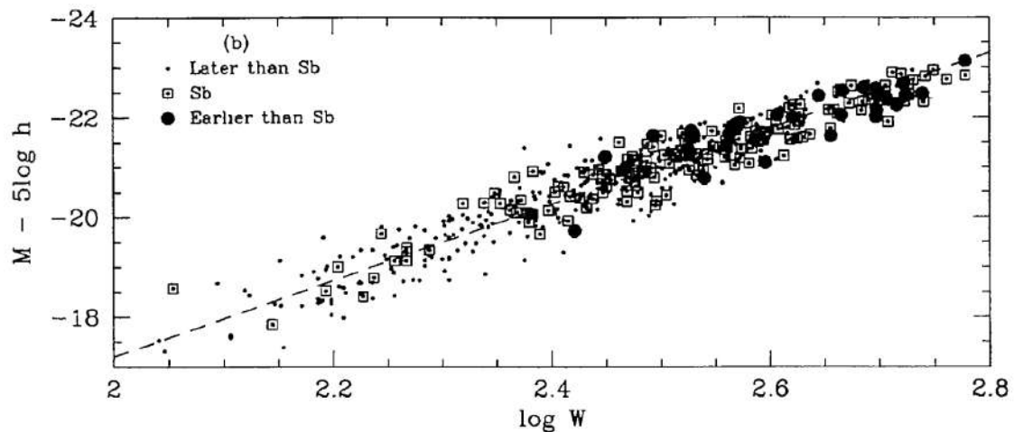
FIGURE 13.13 – Relation de Tully-Fisher. L'axe horizontal est la largeur de raie W , correspondant approximativement au double de v_{\max} , et l'axe vertical représente la magnitude absolue, corrigée de l'expansion de l'Univers. Figure issue de [135].
