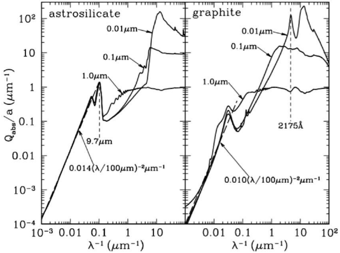
FIGURE 10.18 – Efficacités d'absorption. Elles sont rapportées au rayon a (équivalentes à la section efficace rapportée au volume du grain), pour les silicates et les grains carbonés de différentes tailles (0.01 à 1 \mu\text{m} . Figure issue de [3].
