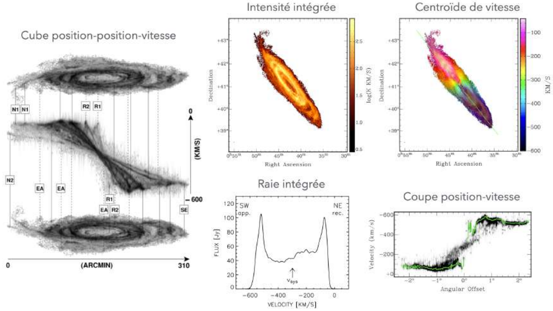
FIGURE 13.11 – Cinématique du HI dans M31. Figure adaptée de [132].
