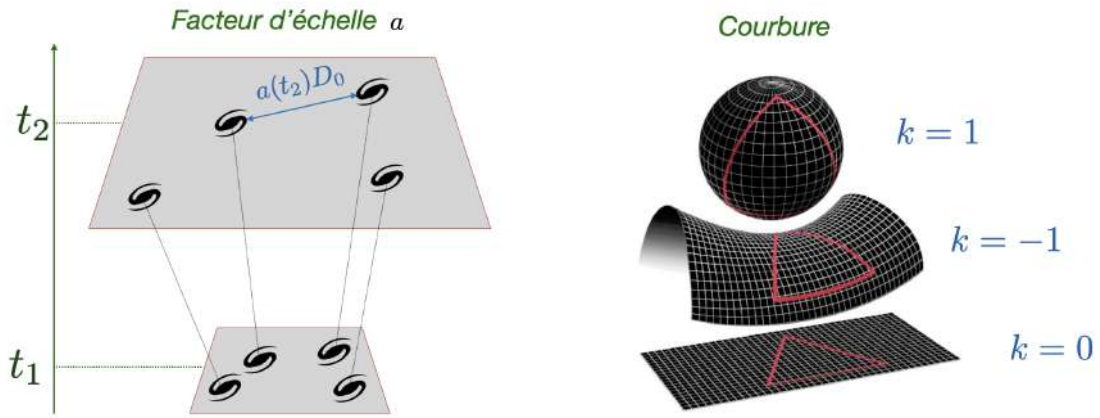
FIGURE 14.5 – Facteur d'échelle et courbure.
