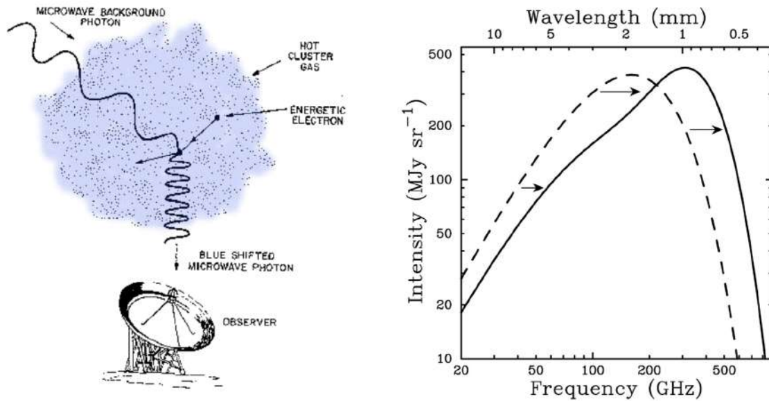
FIGURE 2.14 – Effet Sunyaev-Zel'dovich . Le schéma de gauche présente le principe de l'effet (Crédit : L. Van Speybroeck) et la figure de droite montre la déformation du spectre du CMB (en tirets) par l'effet SZ (traits plein) [17].
