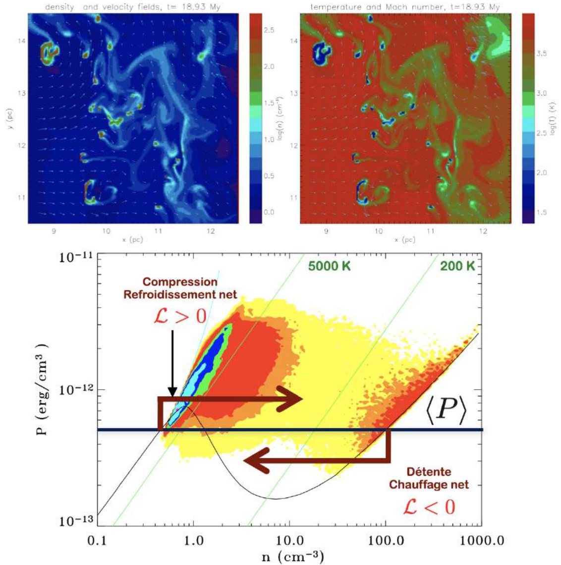
FIGURE 10.16 – Simulation numérique bidimensionnelle de l'instabilité thermique du H I. Champ de densité n_{\text{H}} et de température T et distribution de (n_{\text{H}}, P) dans la simulation. Figure adaptée de [55].
