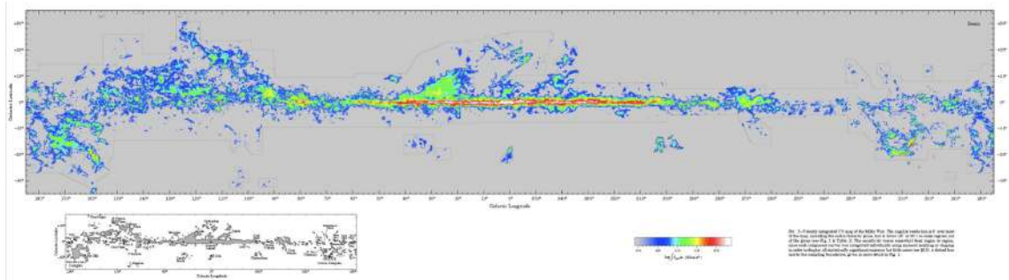
FIGURE 4.10 – Emission CO ( J = 1 \rightarrow 0 ) au voisinage du plan Galactique . Figure issue de [26].
