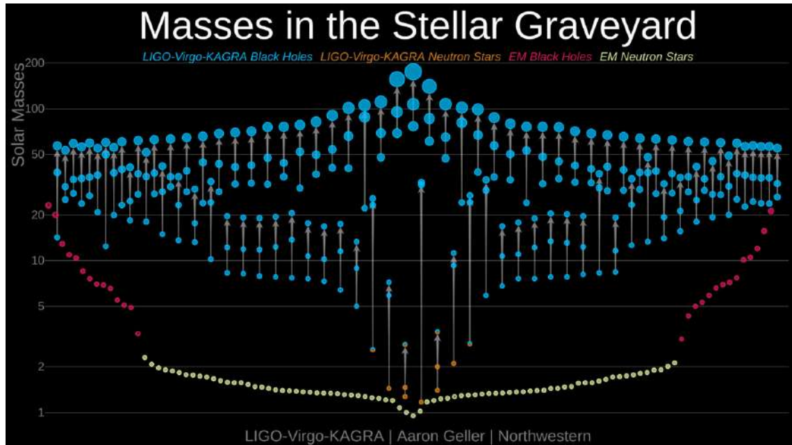
FIGURE 6.4 – Évènements de coalescence détectés avec LIGO-Virgo-KAGRA. Ce graphique montre les masses de toutes les binaires compactes détectées par les instruments LIGO/Virgo/KAGRA, trous noirs (en bleu) et étoiles à neutrons (en orange). Les trous noirs et les étoiles à neutrons détectés en ondes électromagnétiques sont représentés en rouge et en jaune, respectivement.
