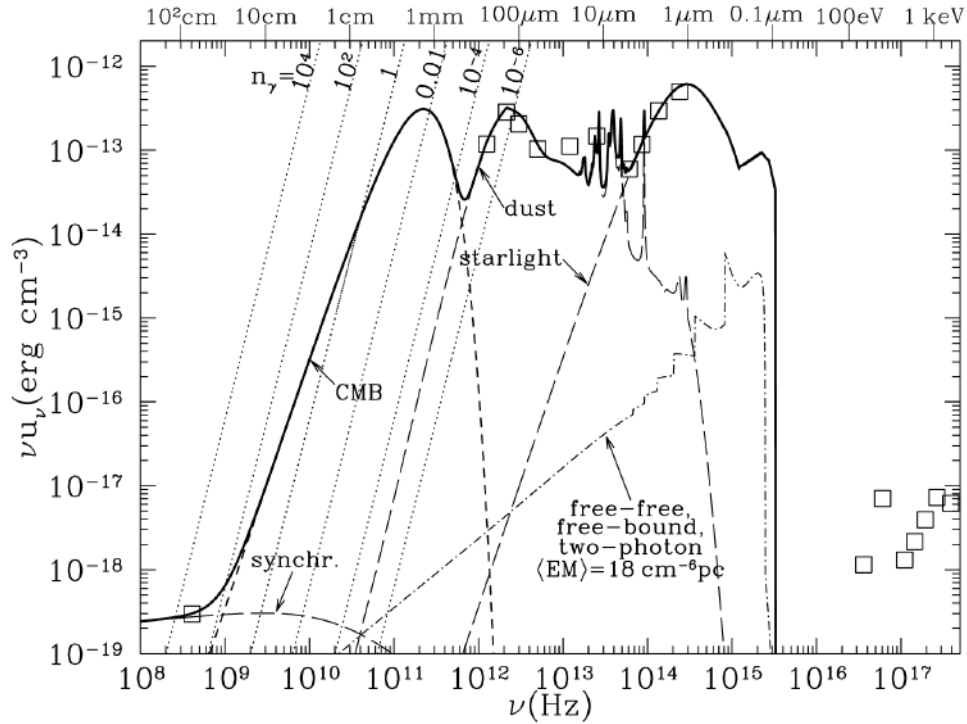
FIGURE 10.25 – Les composantes du champ de rayonnement interstellaire [3].
