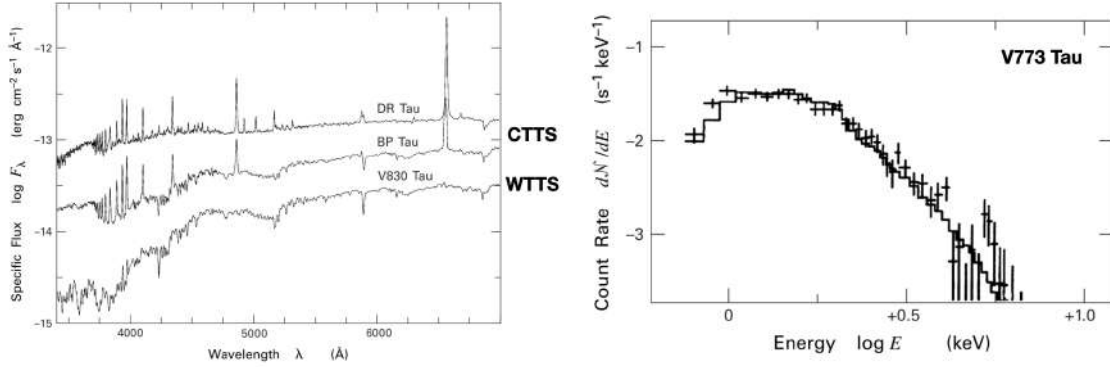
FIGURE 11.7 – Spectres UV-visible de trois T Tauri. On présente le cas des deux T Tauri classiques (CTTS) DR Tau et BP Tau, et de la T Tauri à raies faibles (WTTS) V830 Tau (à gauche) et émission X de la WTTS V773 Tau (à droite). Figure adaptée de [25].
