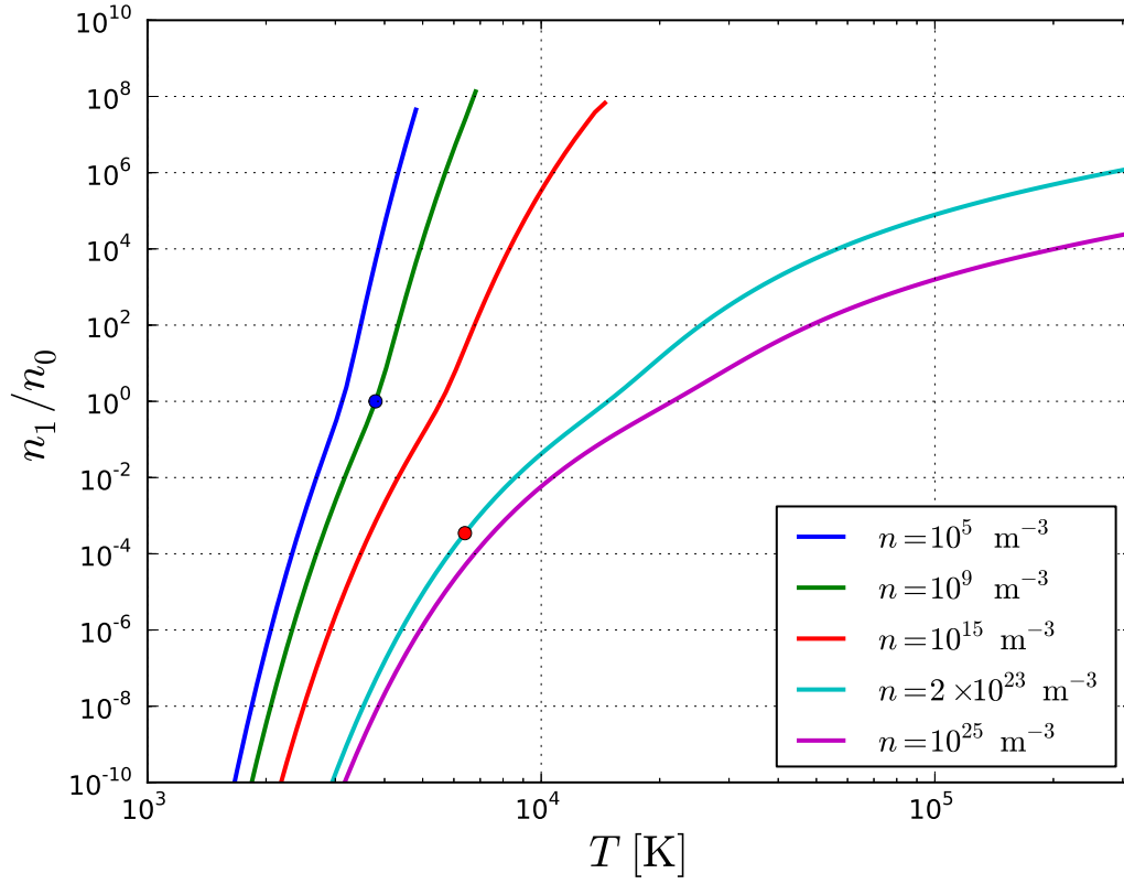
FIGURE 14.12 – Rapport n_1/n_0 = n(\text{H}^+)/n(\text{H}) d'un plasma d'hydrogène en fonction de la température, pour plusieurs densités totales n = n_{\text{H}} . Le cas de la photosphère Solaire ( T = 6400 \text{ K} ) est représenté par le point rouge, celui du découplage ayant donné naissance au CMB par le point bleu.
