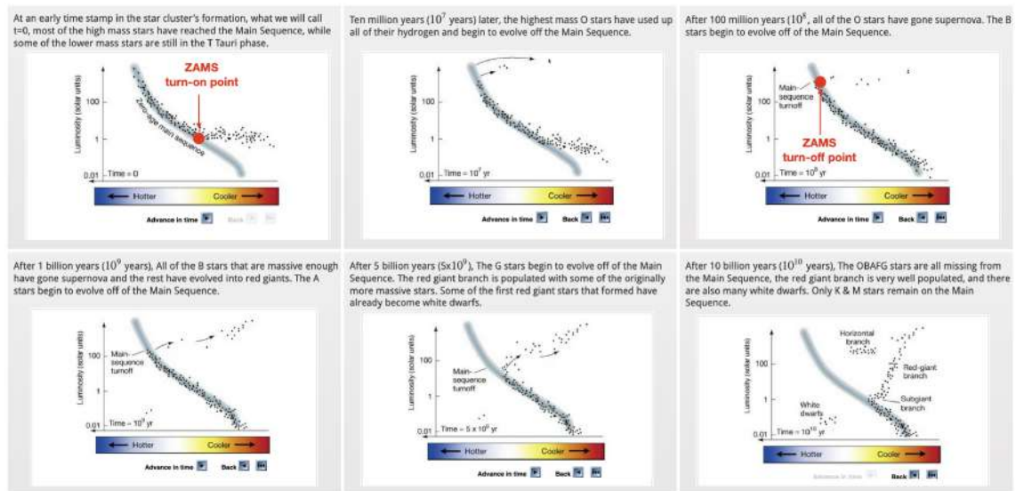
FIGURE 11.10 – Evolution d'une population stellaire dans le diagramme HR. On y voit les "turn-on" et "turn-off" de la séquence principale. Figure adaptée de Penn State Astronomy & Astrophysics ( https://www.e-education.psu.edu/astro801/content/17_p6.html ).
