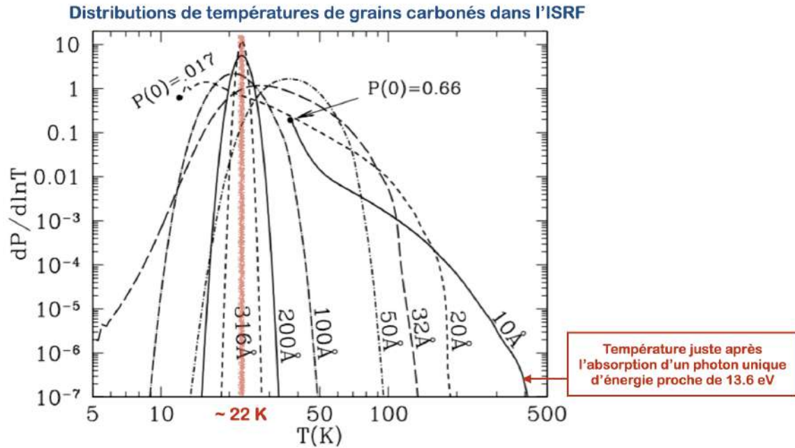
FIGURE 10.22 – Distribution de probabilité des températures de grains. Il s'agit de grains carbonés de différentes tailles. Figure adaptée de [3].
