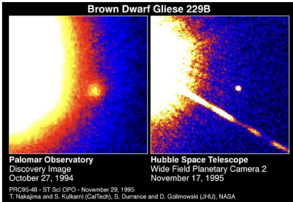
FIGURE 11.33 – Gliese 229B . C'est la seconde naine brune découverte.
