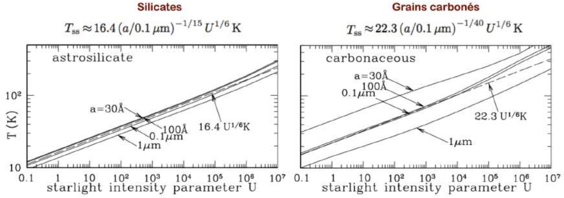
FIGURE 10.20 – Température d'équilibre des silicates et des grains carbonés dans un champ de rayonnement ayant le spectre de l'ISRF, en fonction de l'intensité U du champ, et pour différentes tailles de grains. Figure adaptée de [3].
