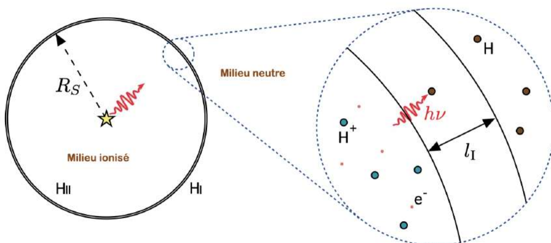
FIGURE 10.12 – Modèle de la sphère de Strömgren.
