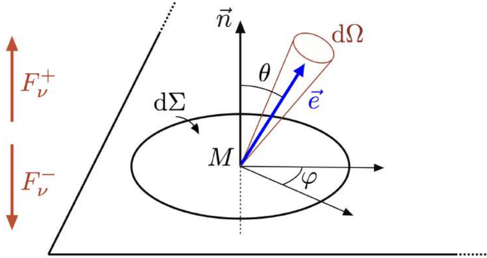
FIGURE 2.3 – Définition des angles \theta et \varphi , et de l'élément d'angle solide d\Omega . Ces notations sont aussi utilisées plus tard pour définir les densités spectrales de flux sortant F_\nu^+ (intégration sur le demi-espace "vers le haut") et entrant F_\nu^- (intégration le demi-espace "vers le bas").
