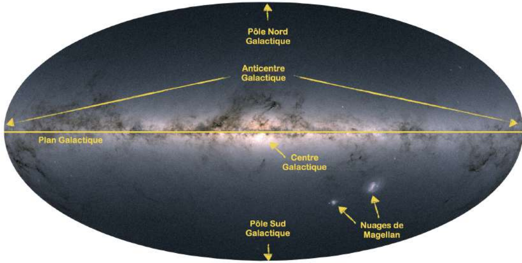
FIGURE 10.28 – Emission visible Galactique observée par Gaia (Crédit : ESA/Gaia/DPAC).
