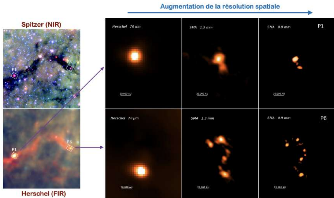
FIGURE 11.32 – Observations de l'IRDC appelé "Nébuluse du Serpent". Avec Spitzer et Herschel à gauche, et avec l'interféromètre submillimétrique SMA à droite (deux dernières colonnes) [91].
