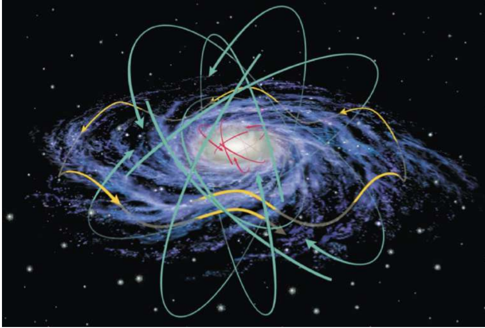
FIGURE 12.20 – Cinématique des étoiles du disque, du bulbe et du halo.
