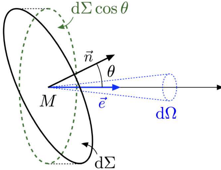
FIGURE 2.2 – Définition de l'intensité spécifique dans une direction quelconque. Notations utilisées pour définir l'intensité spécifique dans une direction \vec{e} quelconque.
