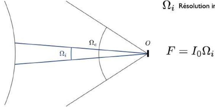
FIGURE 2.6 – Observation d'une source résolue ou non.
