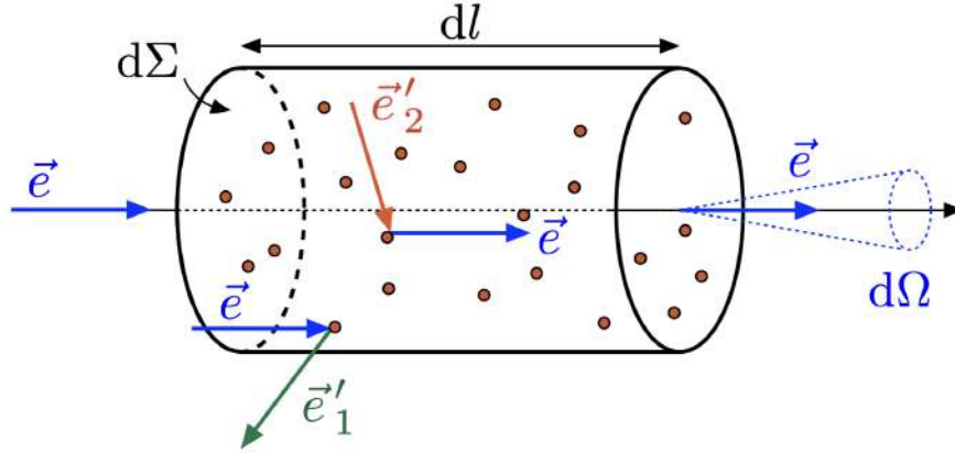
FIGURE 2.16 – Le double effet de la diffusion. La diffusion a pour effet d'une part d'envoyer des photons ayant la direction incidente considérée \vec{e} vers une autre direction \vec{e}'_1 (contribution négative à d\mathcal{E}_\nu ) et d'autre part de ramener dans la direction \vec{e} des photons arrivant dans l'élément de volume dV avec des directions de vol telles que \vec{e}'_2 (contribution positive à d\mathcal{E}_\nu ).
