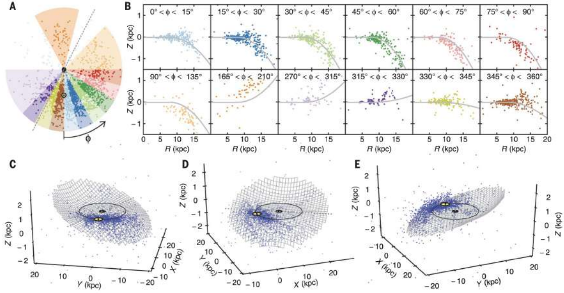
FIGURE 12.7 – Gauchissement du disque stellaire Galactique. Le panneau A montre les positions stellaires projetées dans le plan Galactique, en soulignant différentes régions de longitudes Galactiques données. Pour ces différents secteurs angulaires, le panneau B montre la position des étoiles par rapport au plan z = 0 en fonction de la distance Galactocentrique R . Un ajustement est fait montrant la déviation de la moyenne. Les panneaux C à E montrent les positions stellaires en 3D, pour trois angles de vue différents. Figures issues de [99].
