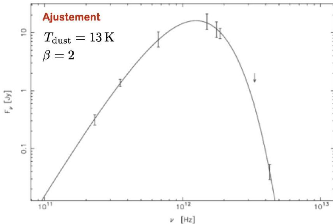
FIGURE 11.16 – Distribution spectrale en  nergie d'un c ur pr stellaire. Ajustement avec une loi de corps noir modifi . Figure adapt e de [80].
