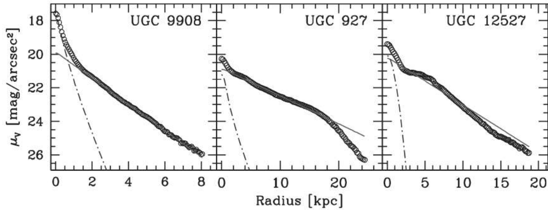
FIGURE 13.6 – Profils de brillance de surface de galaxies spirales.. Figure issue de [131].
