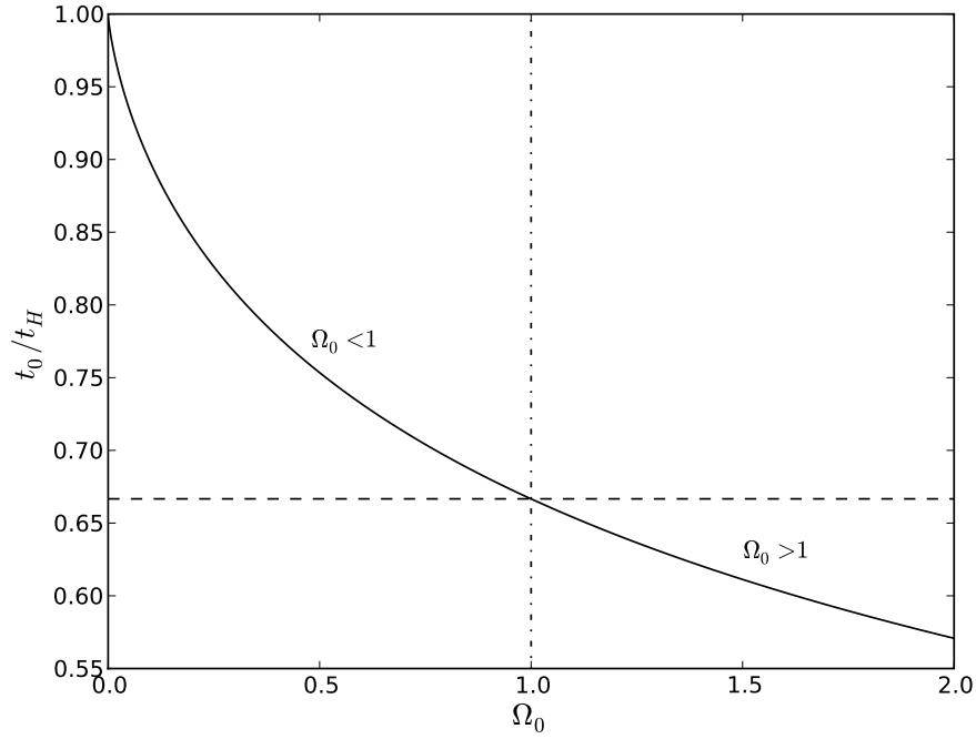
FIGURE 14.6 – Âge calculé pour un Univers poussière de courbure non nulle. L'âge est rapporté au temps de Hubble t_H = 1/H_0 , en fonction du paramètre de densité \Omega_0 . La courbe en tirets marque l'âge calculé dans le cas \Omega_0 = 1 , soit t_0 = (2/3)t_H .
