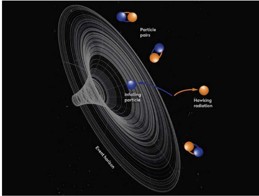
FIGURE 9.6 – Principe du rayonnement de Hawking.
