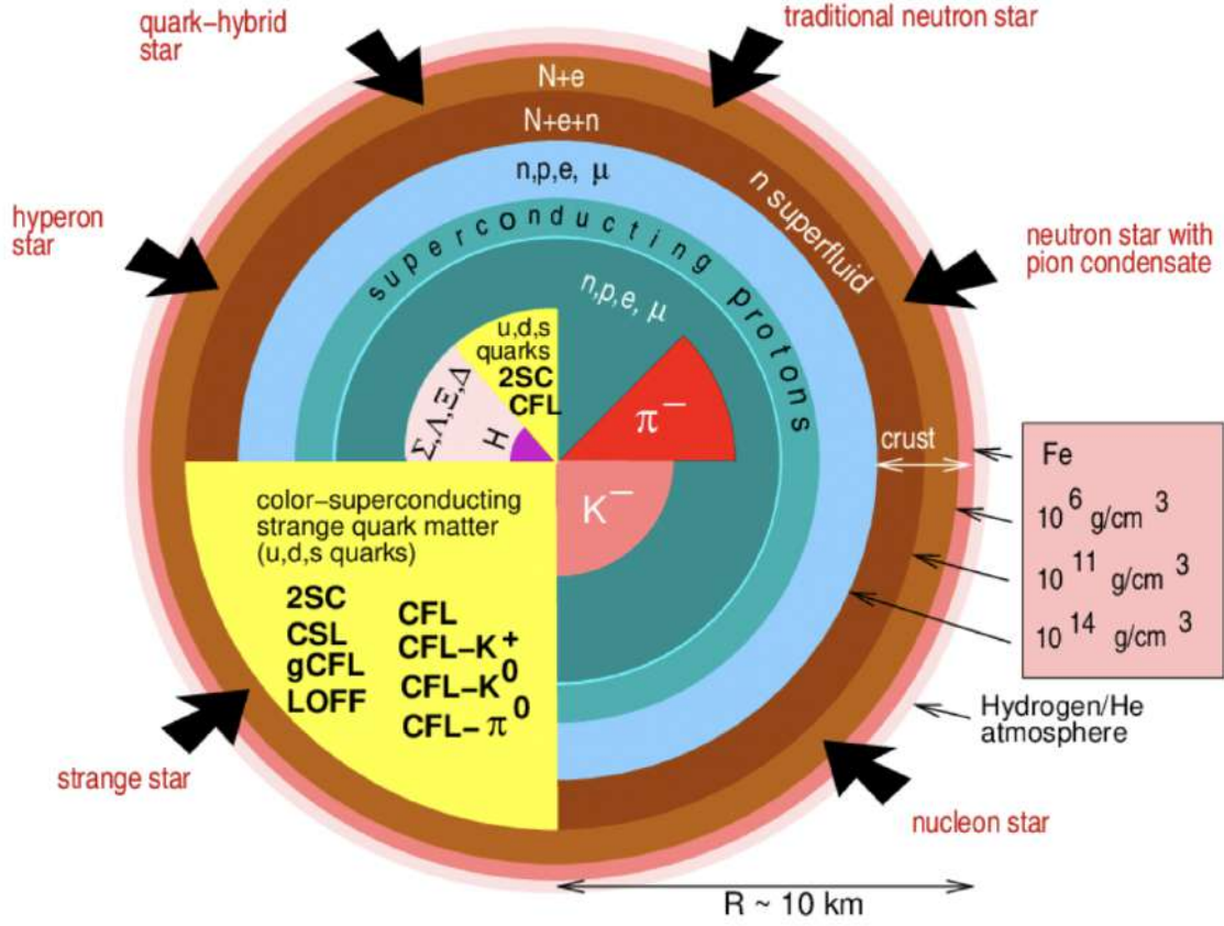
FIGURE 8.1 – Structure d'une étoile à neutrons. Les différents secteurs correspondent à différents modèles d'équations d'état. [Crédit : F. Weber]
