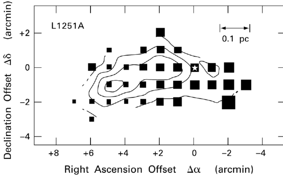
FIGURE 11.21 – Vitesse radiale d'un cœur dense. Cartographie de la vitesse radiale (représentée par la taille des carrés) déduite des mesures de la raie à 1.3 cm de \text{NH}_3 dans le cœur dense L1251A. Figure issue de [25].
