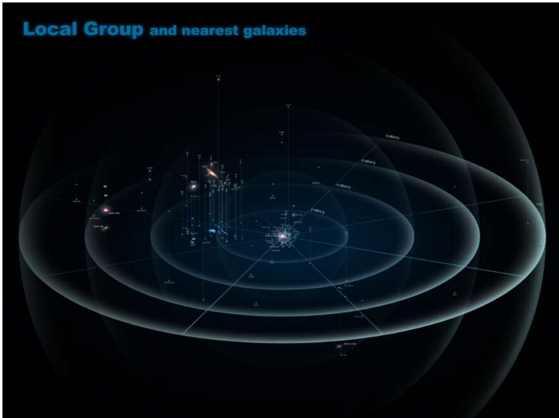
FIGURE 12.23 – Le groupe local (Crédit : A. Ciccolella / Wikimedia Commons)
