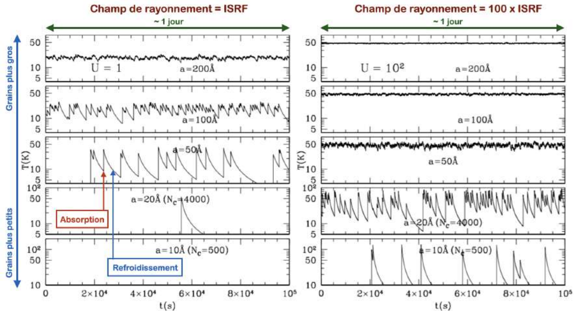
FIGURE 10.21 – Évolution de la température de grains. Des grains de différentes tailles (de plus en plus petits de haut en bas) sont modélisés, pendant une journée environ, dans un environnement correspondant à l'ISRF ( U = 1 , à gauche) ou beaucoup plus intense ( U = 100 , à droite). Figure adaptée de [3].
