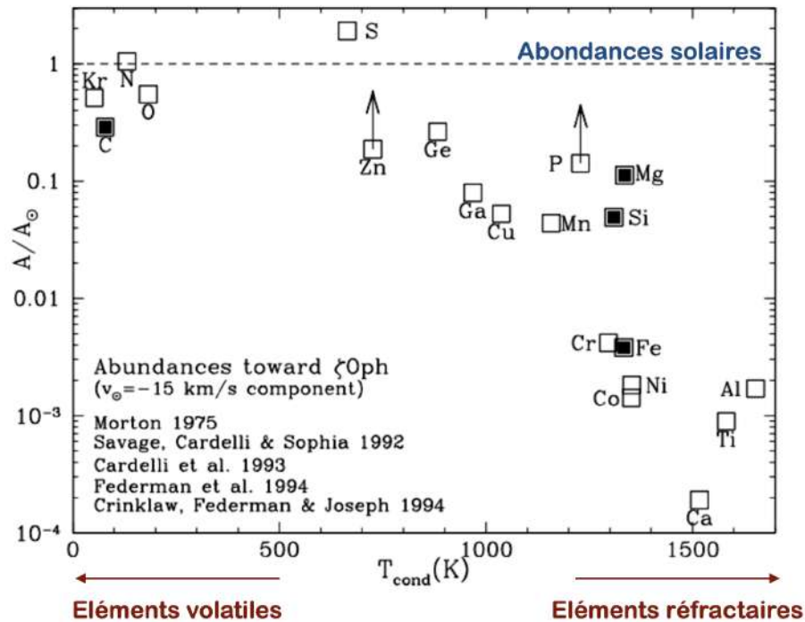
FIGURE 10.23 – Déplétion des éléments en phase gaz. Adapté de [3].
