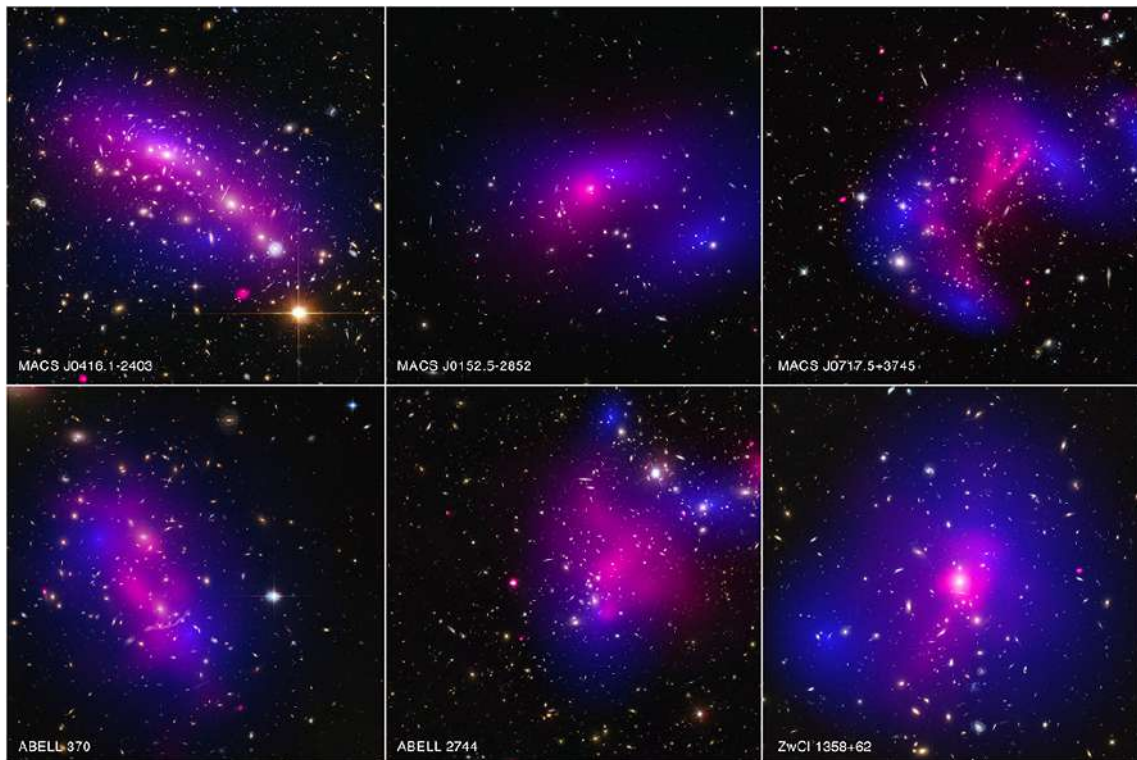
FIGURE 13.26 – Exemples d'amas de galaxies. Aux images en optique obtenues avec HST sont superposées les observations en rayons X (Chandra, en rose) et la distribution de matière totale obtenue par lentillage gravitationnel (en bleu).
