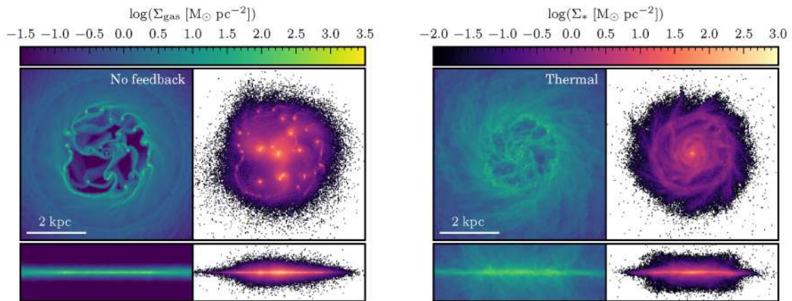
FIGURE 13.24 – La rétroaction des supernovæ. Les deux panneaux montrent la densité surfacique du gaz et celle des nouvelles étoiles, pour une simulation sans feedback (à gauche) et avec une prescription possible de feedback (à droite). Figure issue de [144].
