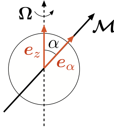
FIGURE 8.4 – Modélisation d'un pulsar. Le moment magnétique dipolaire \vec{\mathcal{M}} fait un angle \alpha avec le vecteur rotation \vec{\Omega} .
