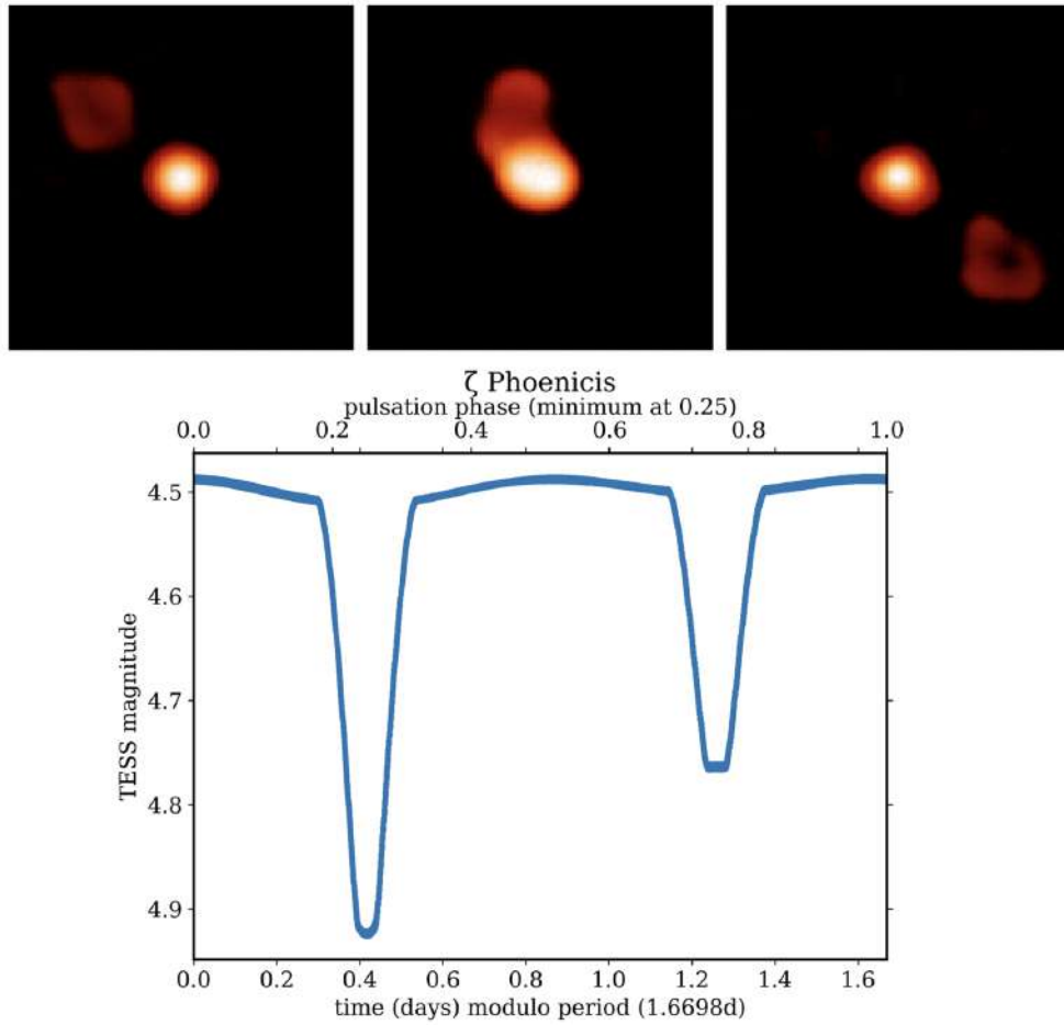
FIGURE 5.9 – Exemple de binaire à éclipse. Les images présentent l’observation de l’éclipse d’Algol B (la plus lumineuse) par Algol A [29]. La figure du bas montre la courbe de lumière (NASA/TESS).
