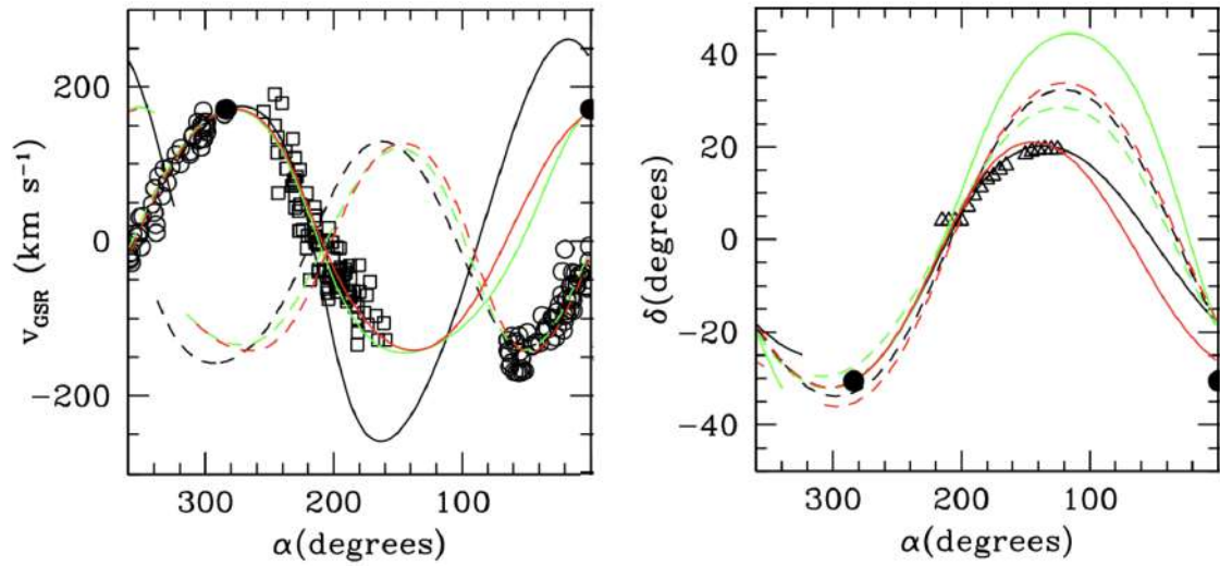
FIGURE 12.16 – Détermination de la forme du halo de matière noire à partir des observations du courant du Sagittaire. Les symboles creux représentent les données de position (à droite) et de vitesse (à gauche) des étoiles du courant du Sagittaire. Le cercle plein représente la position de la galaxie naine du Sagittaire associée à ce courant. Le modèle triaxial permettant de reproduire au mieux les données est représenté par la courbe rouge. Figure issue de [116].
