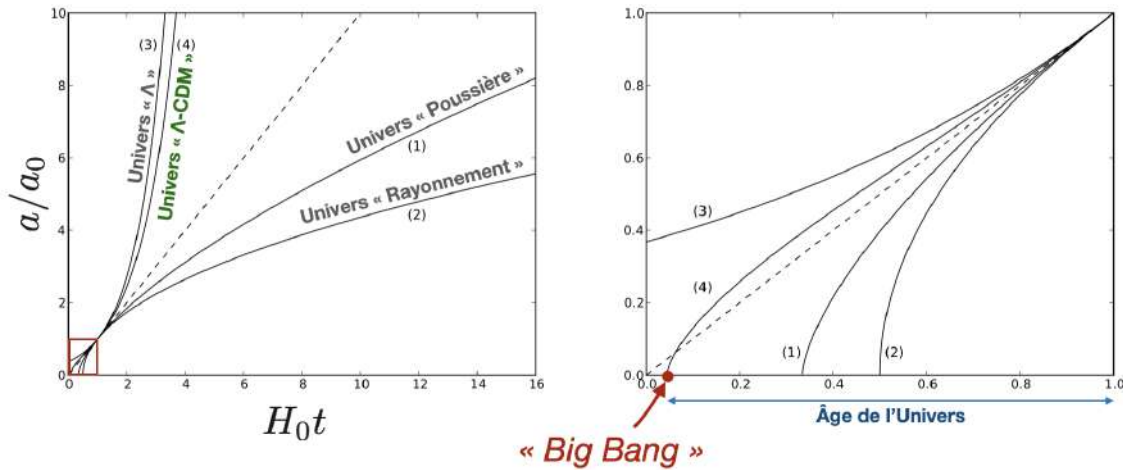
FIGURE 14.7 – Évolution du facteur d'échelle normalisé y = a/a_0 en fonction de x = H_0\tau . Les différents modèles sont présentés avec une origine des temps déplacée pour chaque modèle de façon à ce que les courbes se superposent en x = 1 , pris comme époque actuelle, et ce avec la même pente, imposée par la constante de Hubble H_0 . La droite en pointillés y = x est présentée pour référence. (1) : (\Omega_0 = 1, \omega = 0) (2) : (\Omega_0 = 1, \omega = 1/3) (3) : (\Omega_0 = 1, \omega = -1) (4) : \Lambda -CDM
