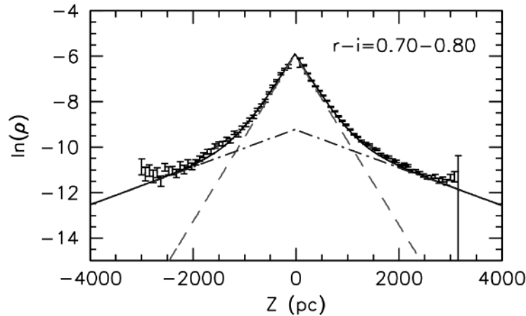
FIGURE 12.5 – Distribution verticale des étoiles de la Galaxie. Les deux contributions des disques mince et épais sont indiquées en tirets et en traits alternés. Figure issue de [97].
