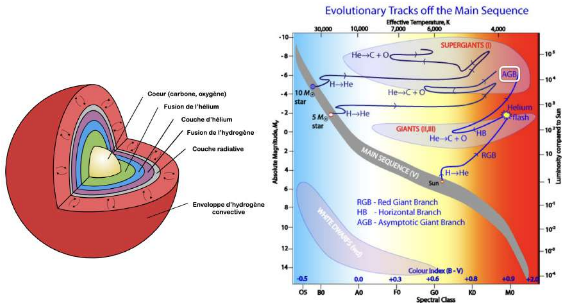
FIGURE 5.26 – Stade AGB. Le schéma de gauche montre la structure d'une telle étoile ( Crédit : M. V. Persson ), celui de droite l'évolution dans le diagramme HR (stade marqué "AGB") ( Crédit : R. Hollow / CSIRO / C. Cain ).
