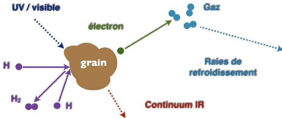
FIGURE 10.17 – Les rôles de la poussière interstellaire.
