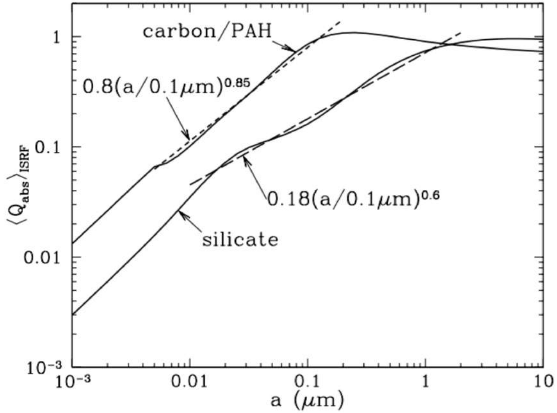
FIGURE 10.19 – Efficacités moyennes d'absorption. Elles sont représentées pour les silicates et les grains carbonés dans l'ISRF de [56] en fonction de leur taille a . Figure issue de [3].
