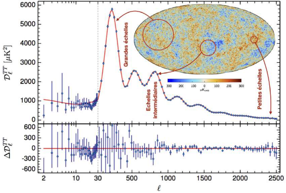
FIGURE 14.14 – Les fluctuations du CMB. La carte en insert représente les fluctuations de température du CMB, de l'ordre de \delta T_{\text{CMB}}/T_{\text{CMB}} \sim 10^{-5} . Leur répartition angulaire est quantifiée par le spectre de puissance représenté par les points de donnée en bleu. Chaque point représente la puissance présente dans le signal à une certaine échelle angulaire \ell , les plus grandes valeurs de \ell correspondant aux plus petites échelles. La courbe en rouge est un ajustement par le modèle \Lambda -CDM à six paramètres . On en tire des valeurs extrêmement précises de ces paramètres, notamment de la constante de Hubble. Figure adaptée de [2].
