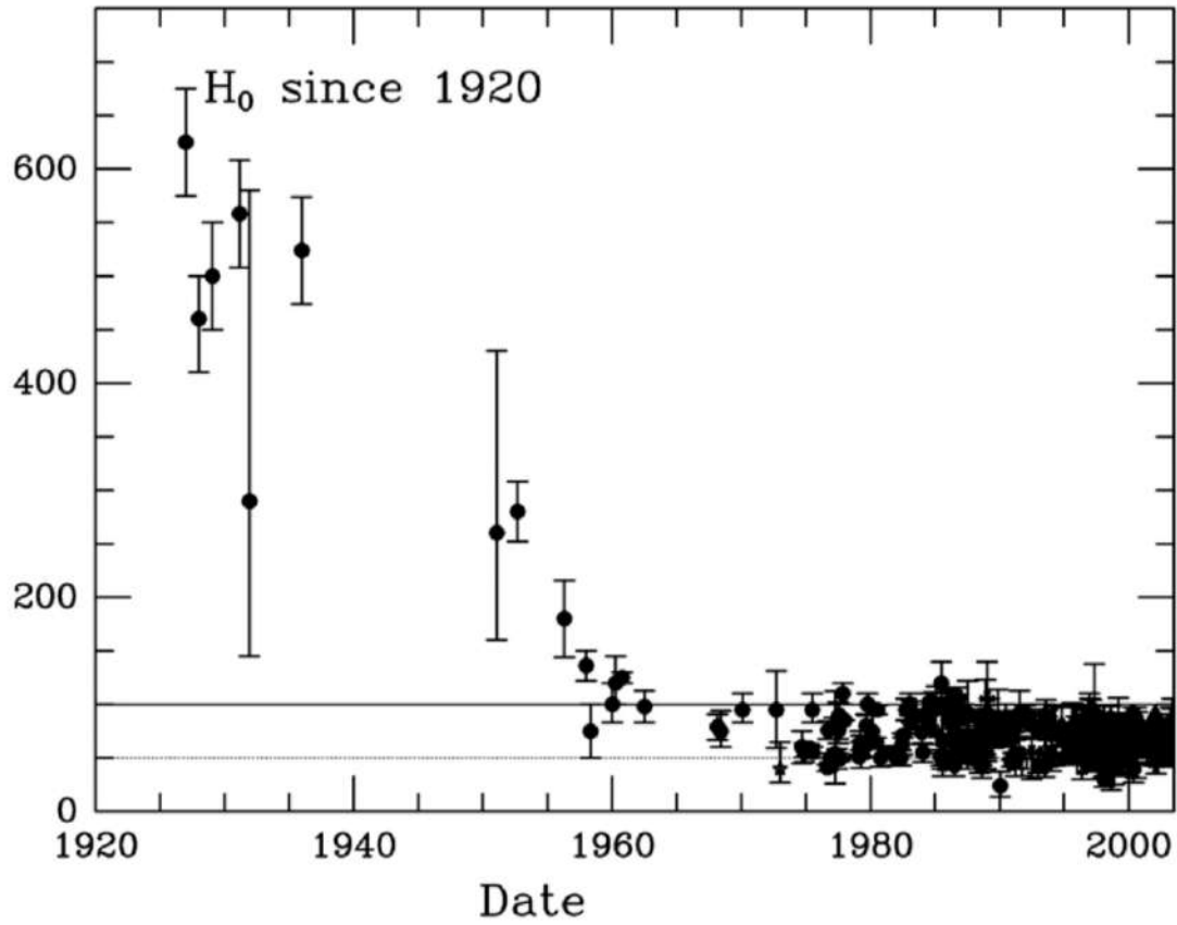
FIGURE 14.3 – Évolution des estimations de la constante de Hubble avec le temps (Source : https://lweb.cfa.harvard.edu/~dfabricant/huchra/hubble/ ).
