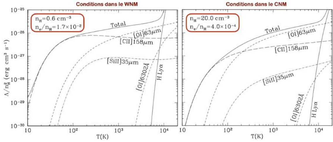
FIGURE 10.14 – Taux de refroidissement \Lambda/n_H^2 en fonction de la température T du gaz. Il est représenté pour des densités n_H et des fractions d'ionisation x_e typiques des conditions dans le WNM (à gauche) et dans le CNM (à droite). Figure issue de [3].
