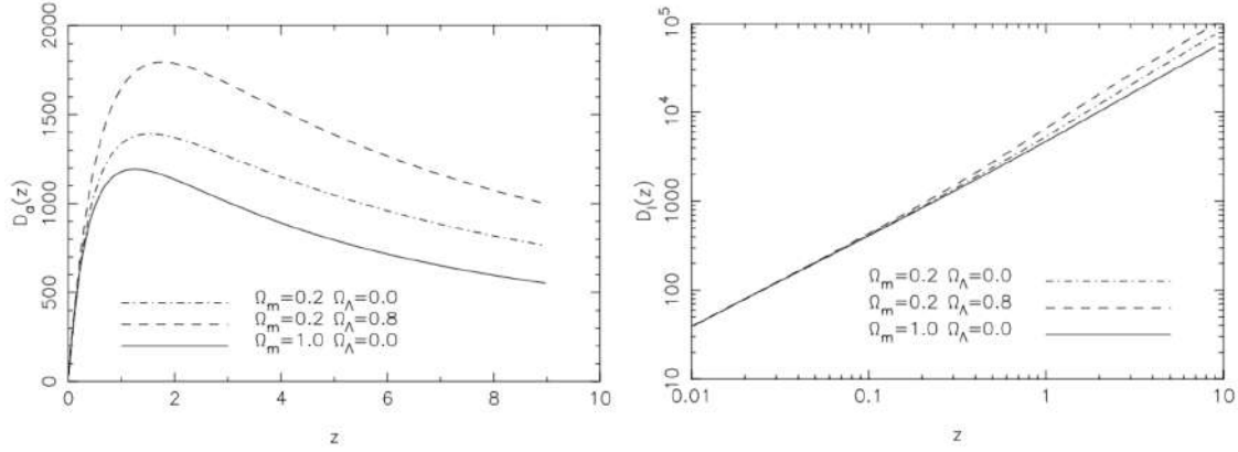
FIGURE 14.10 – Distances angulaire et de luminosité. Les courbes présentent les deux distances en fonction du redshift, pour différents modèles cosmologiques.
