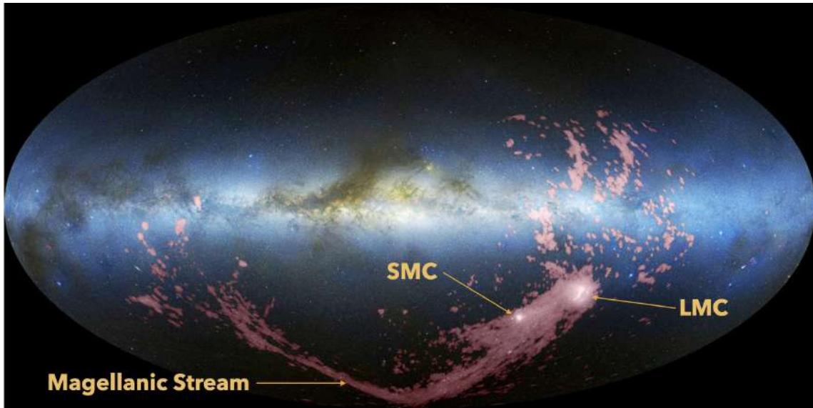
FIGURE 12.24 – Les nuages de Magellan et le courant Magellanique
