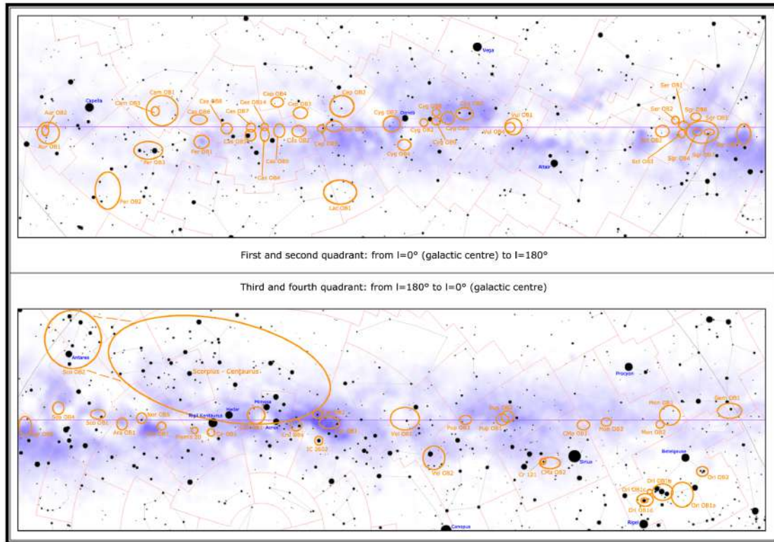
FIGURE 11.2 – Associations stellaires. Les principales associations au voisinage du plan Galactique (R. Mura / Wikipedia).
