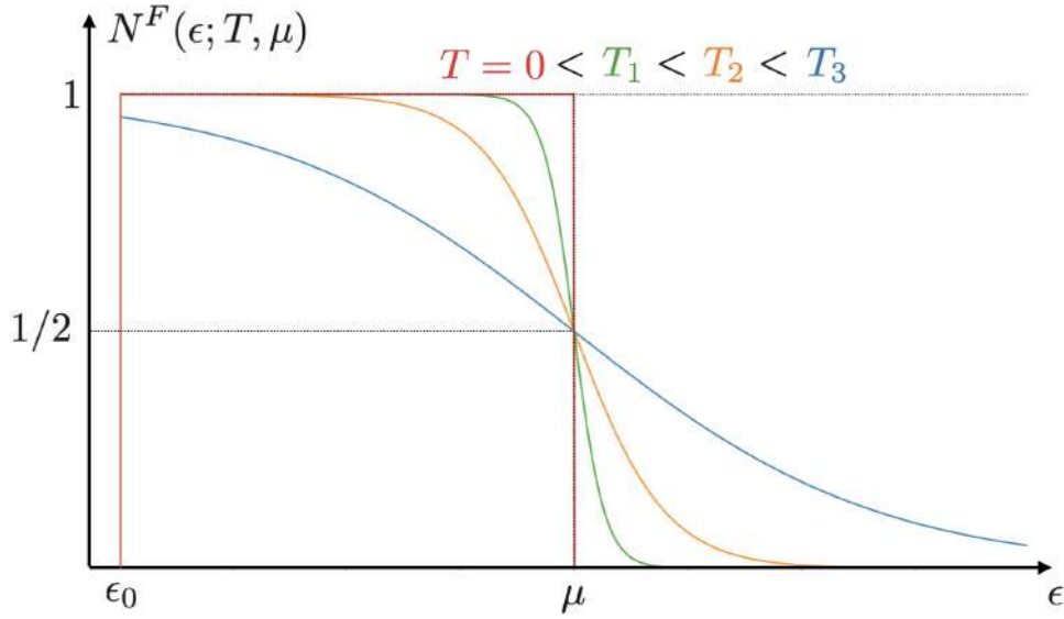
FIGURE 7.2 – Distribution de Fermi-Dirac. La distribution N_{FD}(\varepsilon) est représentée en fonction de l'énergie \varepsilon pour différentes valeurs de la température, y compris T = 0 .
