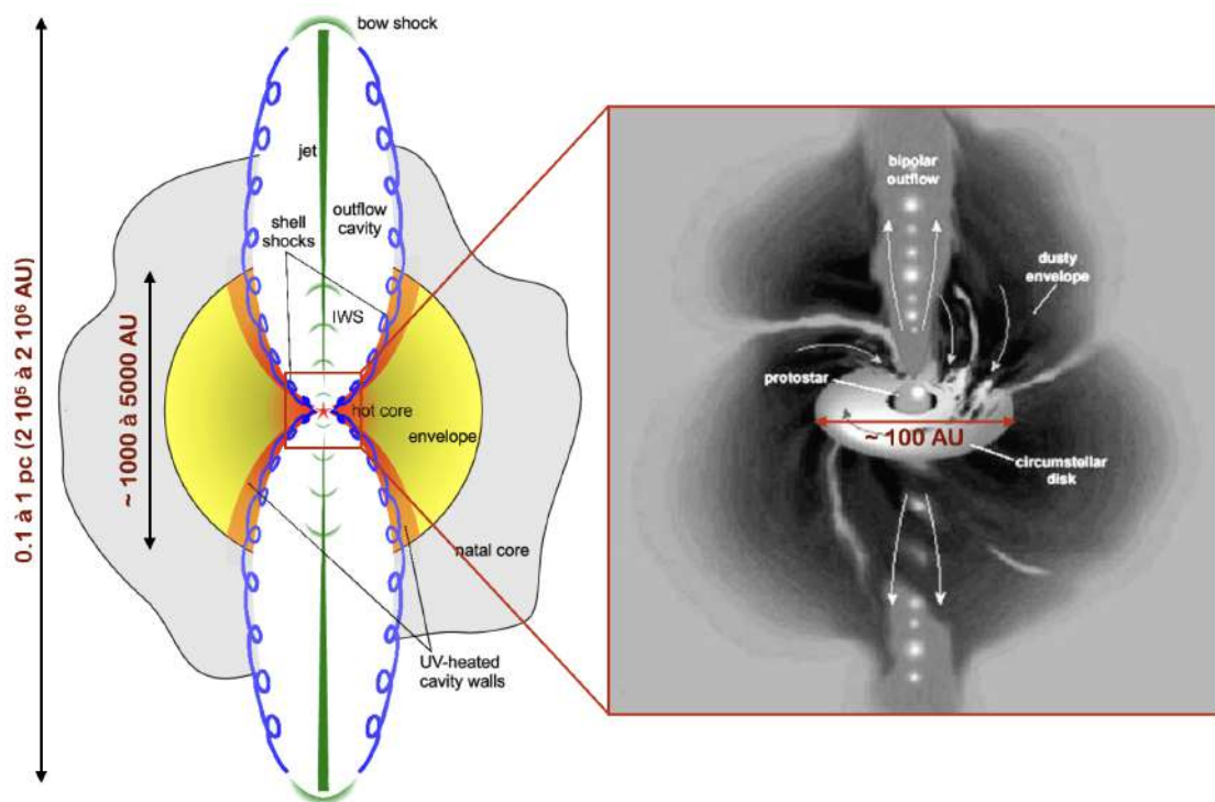
FIGURE 11.30 – Structure d'un objet protostellaire. Figures issues de [90] et https://www.americanscientist.org/article/protostars .
