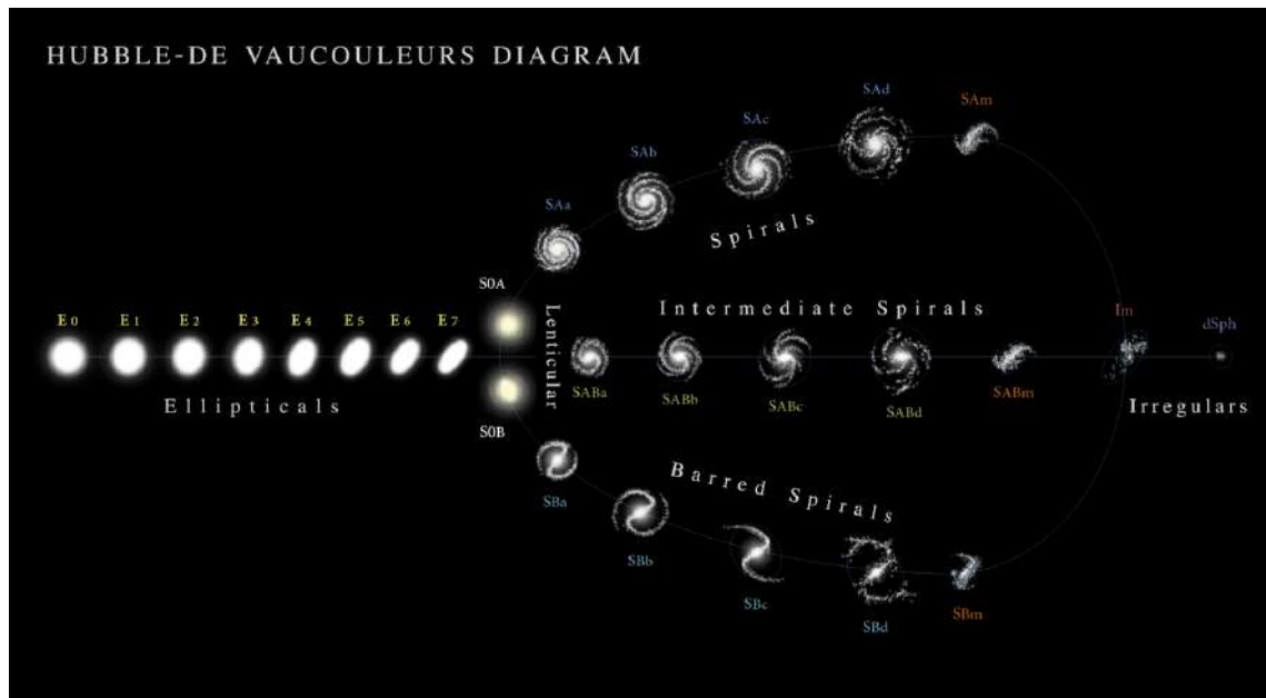
FIGURE 13.1 – Séquence de Hubble-de Vaucouleurs de classification morphologique des galaxies.
