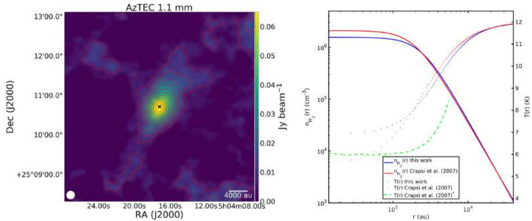
FIGURE 11.15 – Le cœur pr stellaire L1544. Observations millim triques de L1544 (  gauche) et profils de densit  et de temp rature d duits (  droite). Figures issues de [79].
