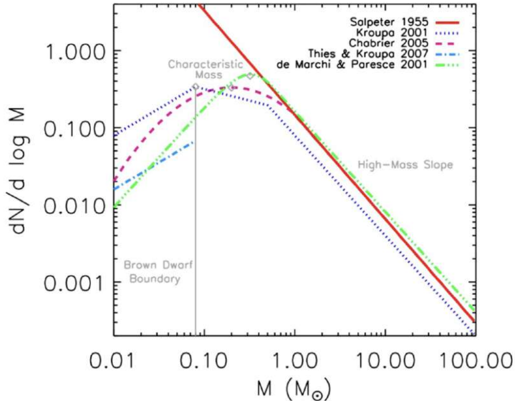
FIGURE 10.3 – Fonction de masse initiale des étoiles [48]. Les différentes courbes correspondent à différents modèles empiriques ou semi-empiriques de l’IMF. Leurs écarts aux faibles masses sont dûs à l’incomplétude des relevés, associée à leur sensibilité limitée.
