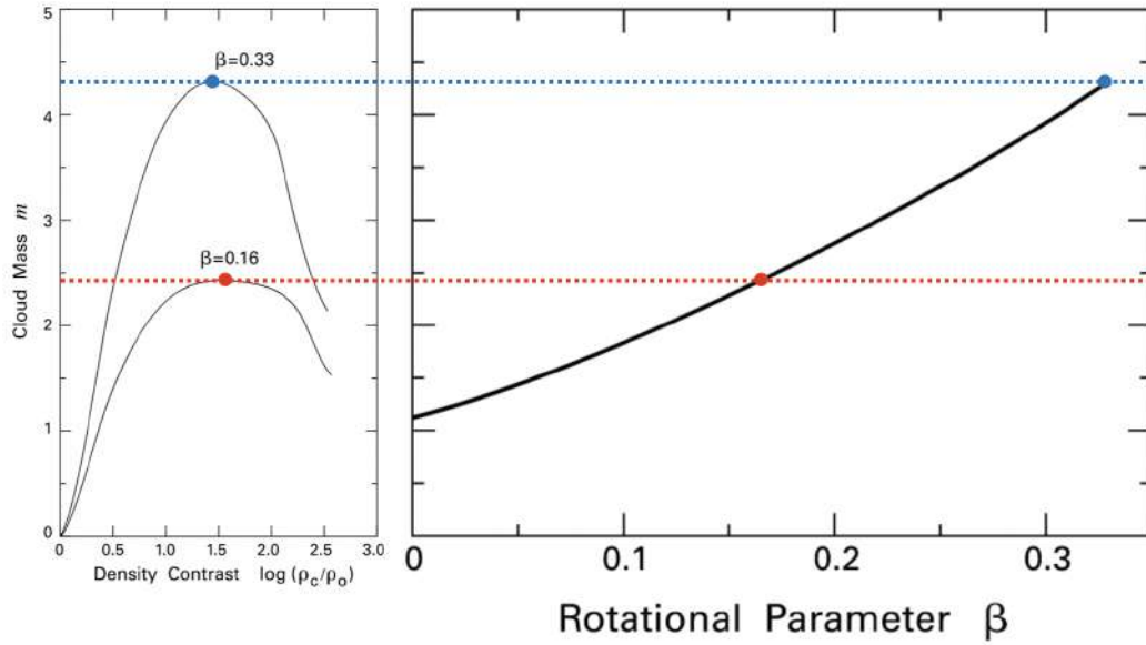
FIGURE 11.20 – Influence de la rotation sur la stabilité. Courbes m(\rho_c/\rho_0) pour deux paramètres de rotation \beta (à gauche) et évolution de la masse critique marquant le premier maximum de m(\rho_c/\rho_0) , en fonction de \beta (à droite). Figures adaptées de [25].
