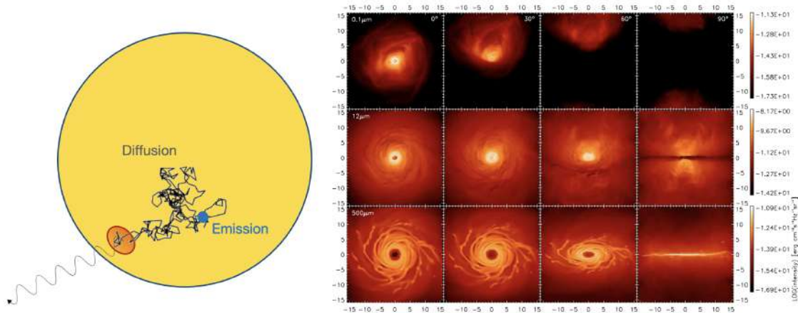
FIGURE 2.17 – Marche au hasard et méthodes Monte Carlo. Le schéma de gauche montre une marche au hasard d'un photon émis à l'intérieur du Soleil et diffusé de nombreuses fois avant d'être émis à la surface. La figure de droite montre le résultat d'observations synthétiques avec le code de transfert radiatif Monte Carlo RADMC-3D sur des simulations d'un tore poussiéreux autour d'un noyau actif de galaxie [18].
