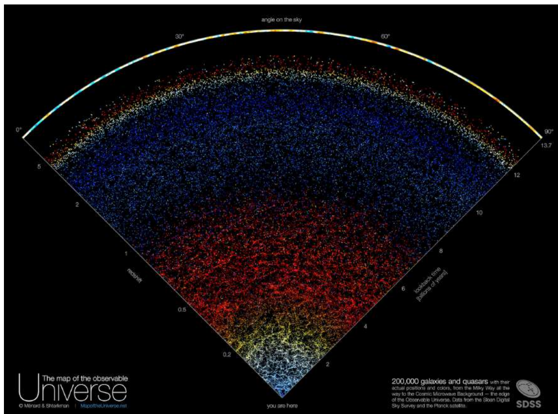
FIGURE 13.2 – Le relevé spectroscopique SDSS. Chaque point correspond à une galaxie, et la couleur en traduit le redshift.
