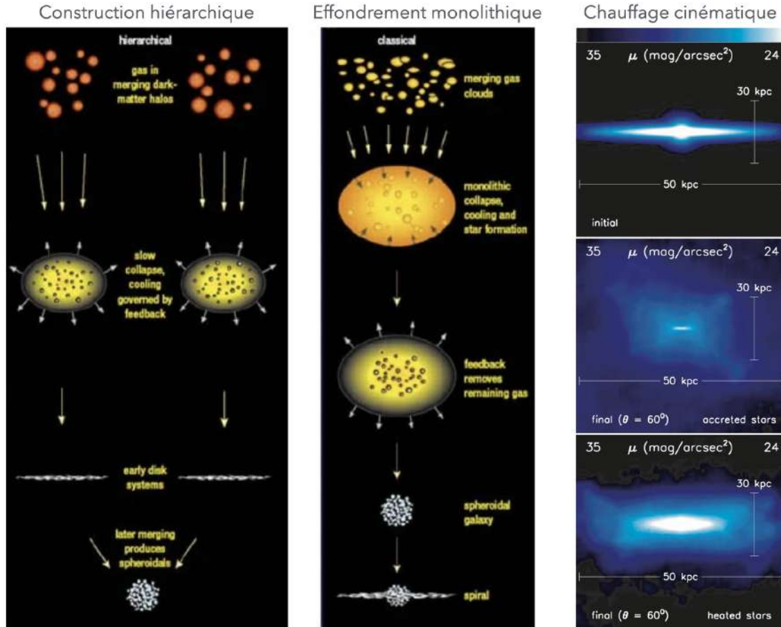
FIGURE 12.11 – Scenarii de formation du halo stellaire. Le panneau de gauche présente le cas de la construction hiérarchique, celui du milieu le cas de l'effondrement monolithique et celui de droite montre une simulation du scénario de chauffage cinématique du disque [108], avec le disque initial en haut, les étoiles du satellite accréte au milieu et les étoiles du disque chauffées en bas.
