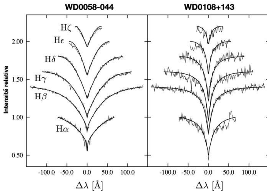
FIGURE 7.7 – Raies de Balmer de naines blanches . Chaque figure correspond à une naine blanche, et représente les raies de Balmer H\alpha à H\zeta (décalées en ordonnées pour une meilleure visibilité) observées dans le spectre de ces étoiles, avec des ajustements (traits épais) permettant de contraindre simultanément la gravité de surface et la température effective. Figure adaptée de [40].
