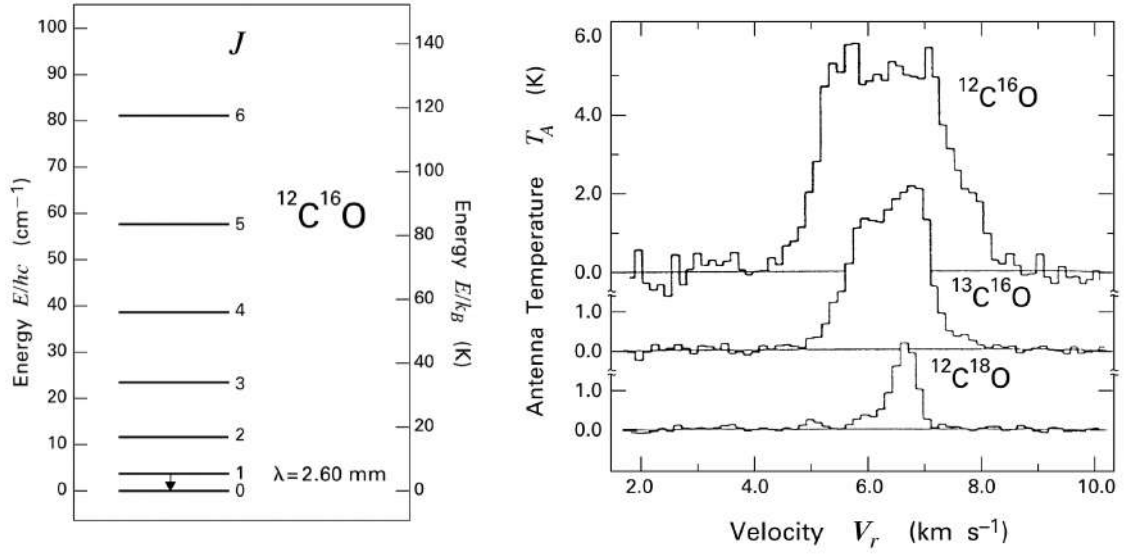
FIGURE 4.9 – La molécule CO . Niveaux rotationnels (à gauche) et profils de raies J = 1 \rightarrow 0 d'isotopologues de CO observés en direction du complexe moléculaire Taurus-Auriga. Figures issues de [25].
