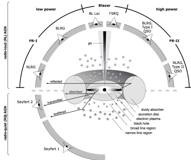
FIGURE 6.6 – Modèle unifié des AGN. Figure issue de [36].
