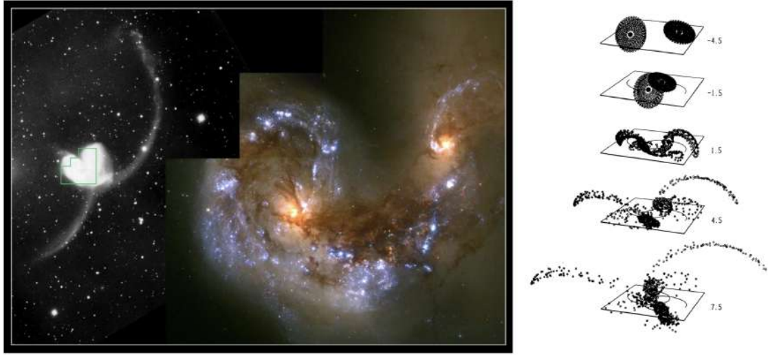
FIGURE 13.20 – Les galaxies des Antennes. Le zoom sur la région centrale montre une grande quantité de poussières et de nombreuses régions de formation stellaire. Le panneau de droite montre l'évolution d'une simulation de ce système (figure issue de [141]).
