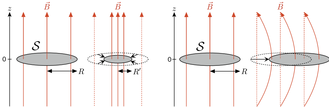
FIGURE 11.22 – Interprétation de la pression et de la tension magnétiques. Sur le panneau de gauche, on considère le cas de la contraction homothétique d'une surface circulaire de rayon initial R , les lignes de champ magnétiques restant parallèles à l'axe Oz . Sur le panneau de droite, on considère le cas où la surface circulaire n'est pas déformée mais se déplace globalement, les lignes de champ restant fixées à grande distance sur l'axe Oz .
