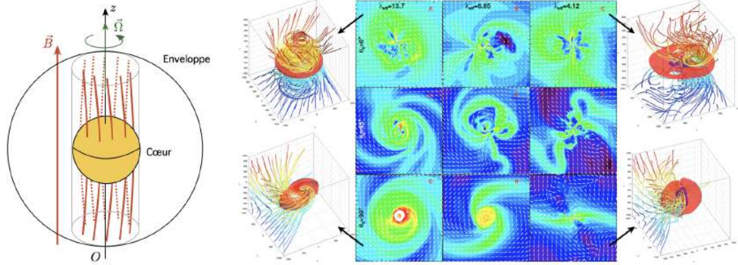
FIGURE 11.25 – Freinage magnétique. Schéma montrant le principe du freinage magnétique par enroulement des lignes de champ, propagation d'ondes d'Alfvén vers l'enveloppe et mise en co-rotation de celle-ci (à gauche) et simulations numériques de cet effet [87].
