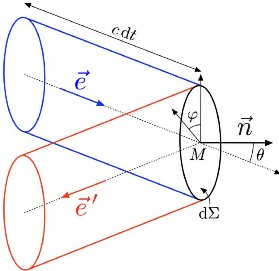
FIGURE 2.7 – Définition de la pression de radiation
