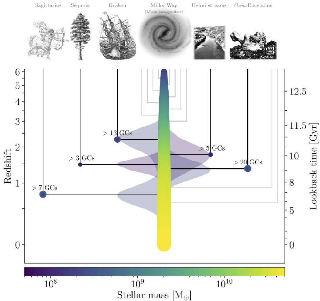
FIGURE 12.22 – Histoire des accrétions majeures de la Voie lactée. Dans cet "arbre généalogique", chaque branche correspond à une galaxie satellite différente accrétée à des époques différentes. Figure issue de [124].
