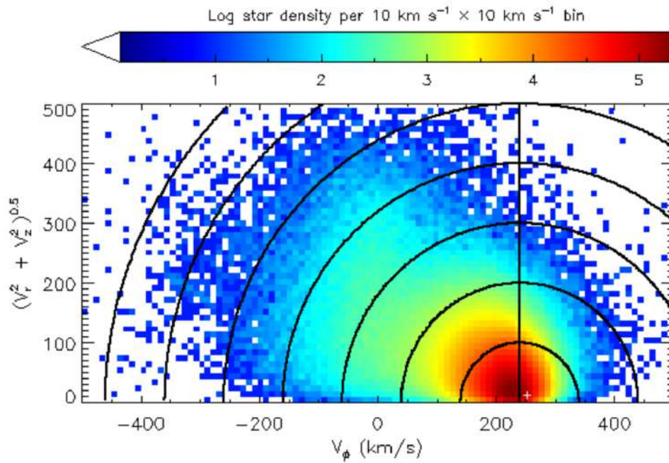
FIGURE 12.21 – Diagramme de Toomre pour \sim 7 millions d'objets dans les données Gaia (DR2).
