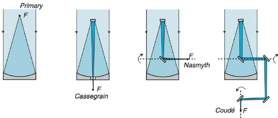
FIGURE 1.11 – Quelques configurations usuelles de télescopes. Le point F est le point focal de la source située à l'infini sur l'axe de pointage du télescope. Figure issue de [8].
