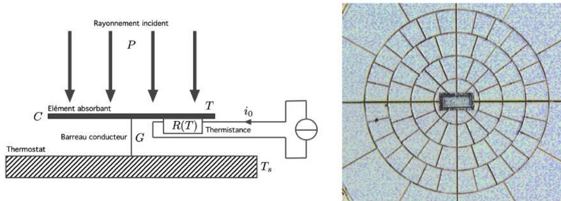
FIGURE 1.17 – Bolomètres . Schéma de principe (à gauche) et exemple d'un bolomètre à 143 GHz de l'instrument HFI sur la mission Planck . L'élément absorbant est la grille qui donne son nom au type de bolomètre, et le dispositif rectangulaire au centre est le circuit de mesure de la température. (Source : https://shorturl.at/jvCG7 ).
