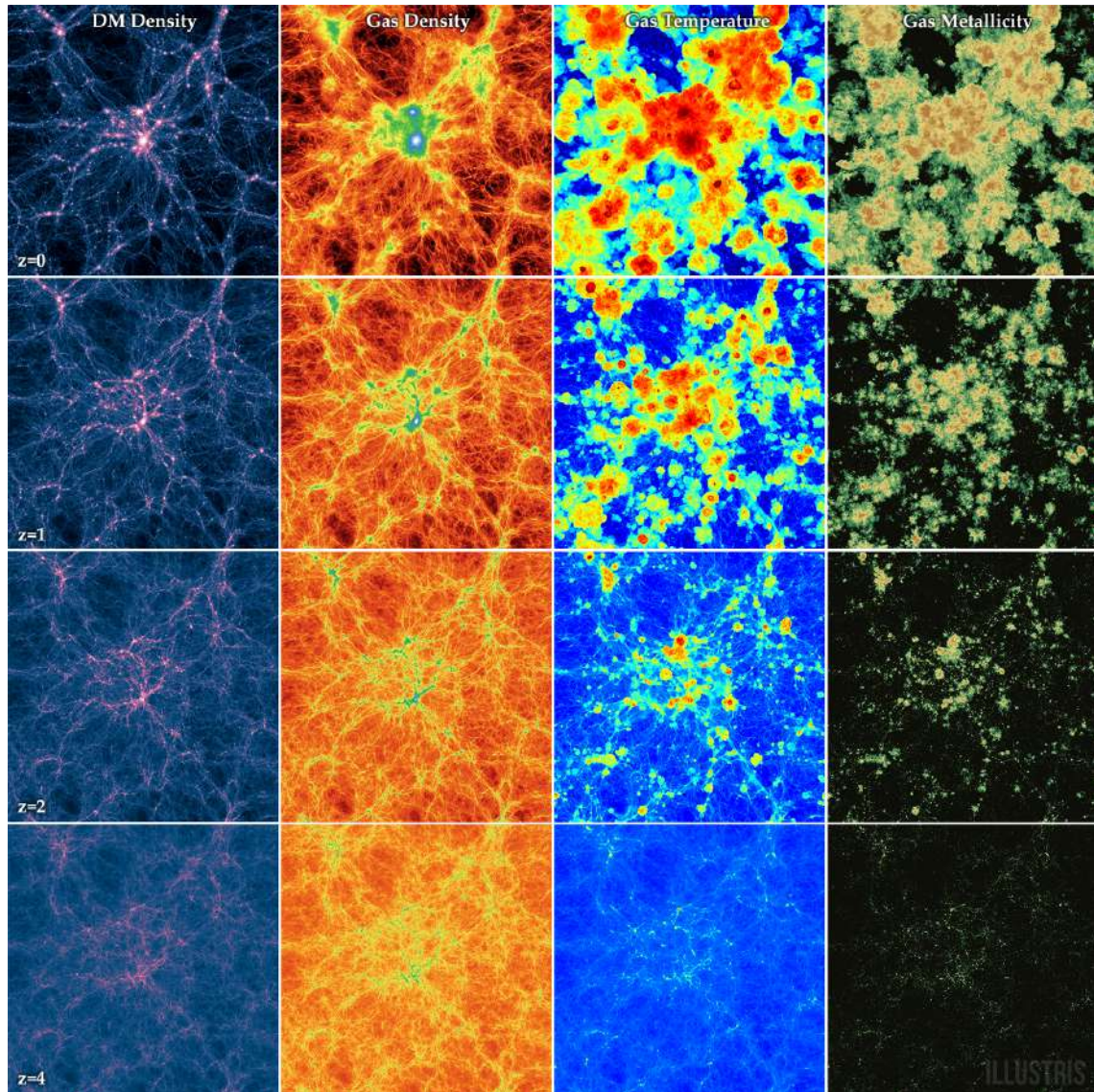
FIGURE 13.29 – Illustris Simulation. Les différents panneaux montrent la distribution de la matière noire, la densité du gaz, sa température et sa métallicité, pour quatre redshifts différents, de z = 4 à z = 0 . Figure issue de https://www.illustris-project.org/ .
