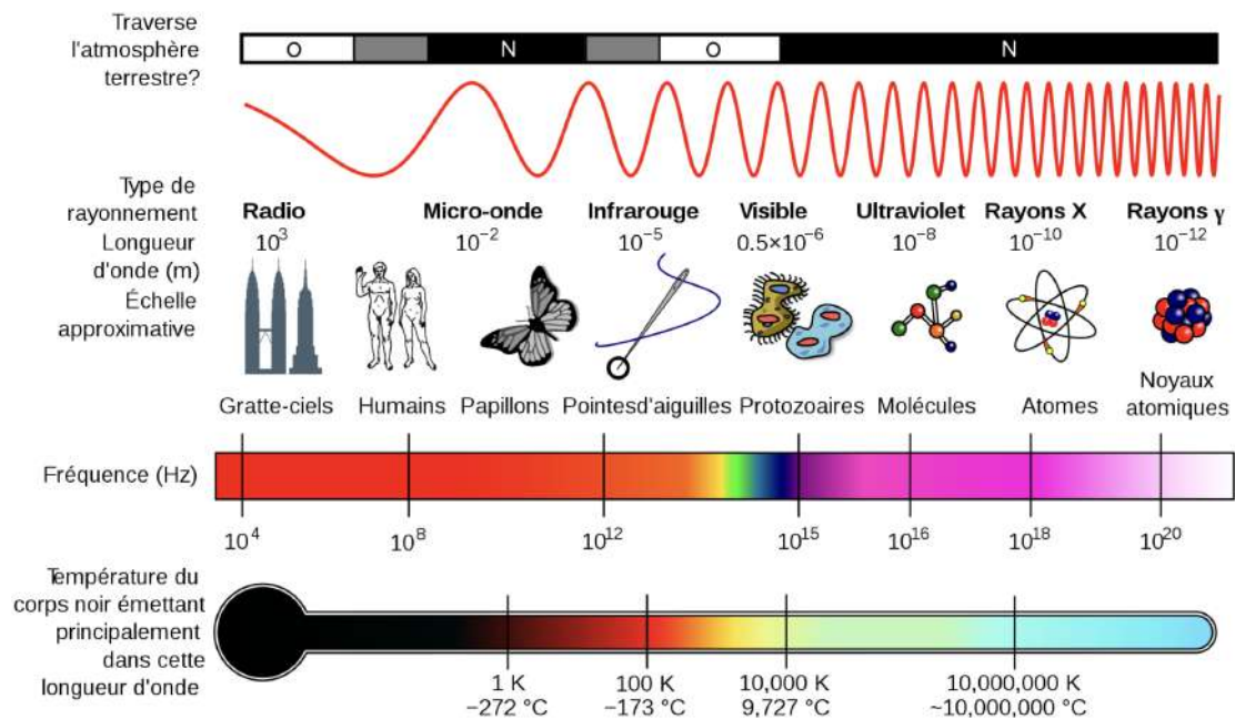
FIGURE 1.1 – Le spectre électromagnétique (Source : Wikimedia Commons)
