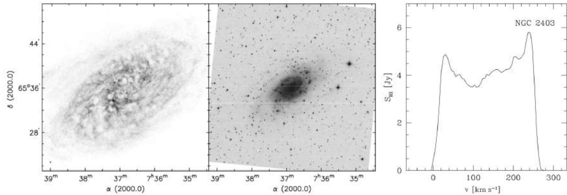
FIGURE 4.8 – Raie à 21 cm de NGC 2403. Intensité intégrée dans la raie (à gauche), image optique issue du DSS (au milieu) et spectre intégré de la raie (à droite) [24].
