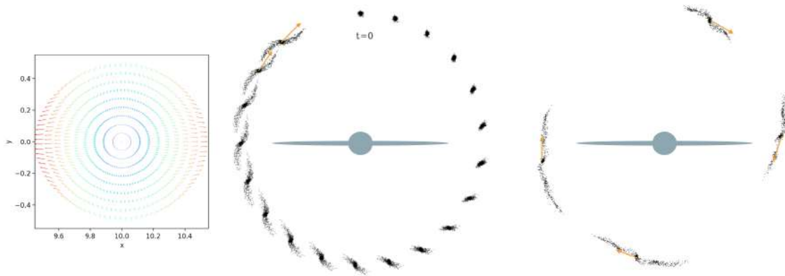
FIGURE 13.19 – Effets de marée. Le panneau de gauche montre le champ de force de marée dans un objet de masse m à la distance R d'un corps de masse M , les deux étant alignés sur l'axe des x , le panneau central et le panneau de droite montrent l'effet au cours du temps de ce champ de marée sur un groupement d'étoiles initialement sphérique en orbite autour d'une galaxie [Crédit : P. Di Matteo].
