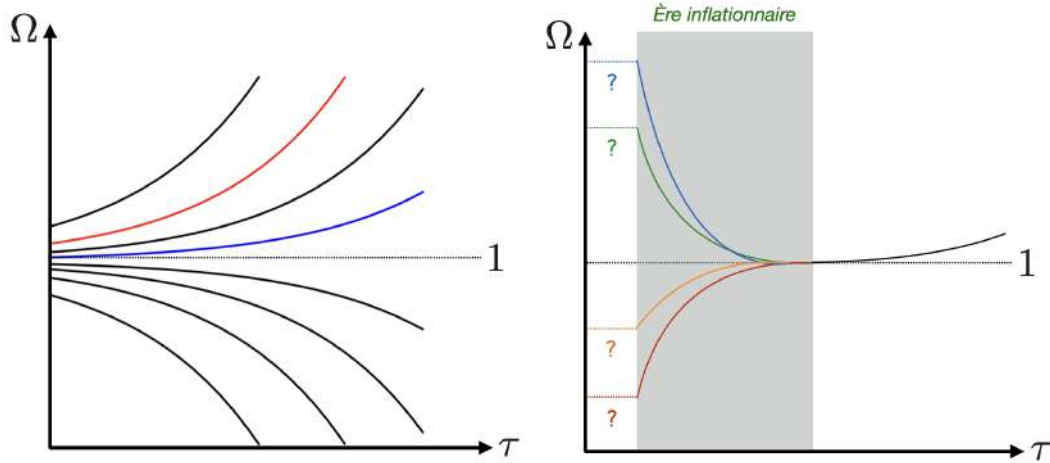
FIGURE 14.15 – Le problème de la courbure . La figure de gauche présente le problème dans le cadre du modèle du Big Bang, et celle de droite présente sa résolution dans le paradigme de l'inflation.
