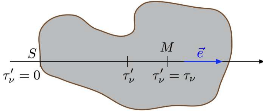
FIGURE 2.10 – Calcul de l'intensité dans un nuage. Pour obtenir la valeur de I au point M , on intègre l'équation du transfert entre S et M avec la condition aux limites I(S, \vec{e}) = I_0 .
