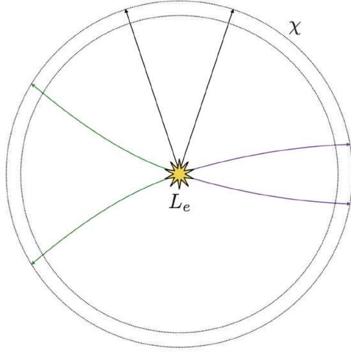
FIGURE 14.9 – La distance apparente de luminosité.
