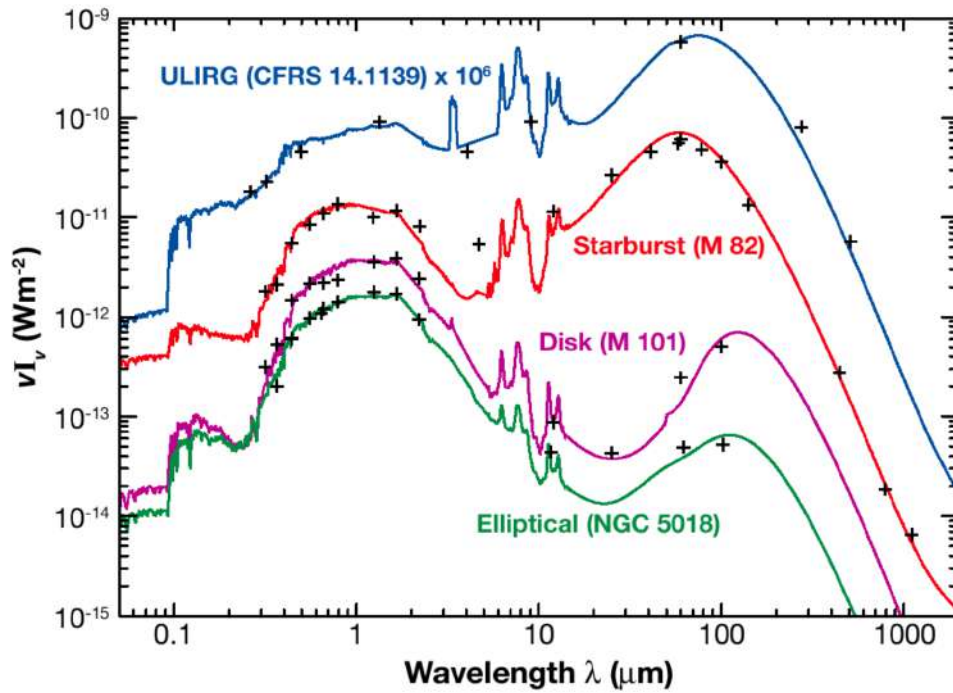
FIGURE 13.21 – Distributions spectrales en énergie de galaxies. Figure issue de [142].
