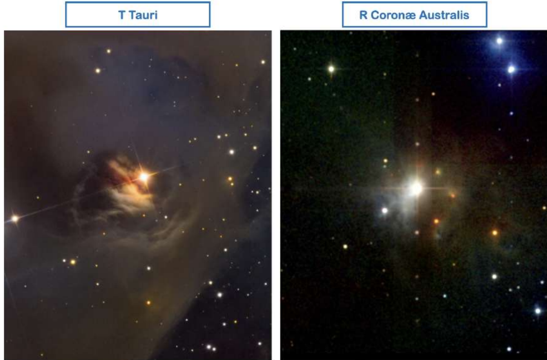
FIGURE 11.6 – Des objets stellaires jeunes. T Tauri (à gauche) et R Coronæ Australis (à droite).
