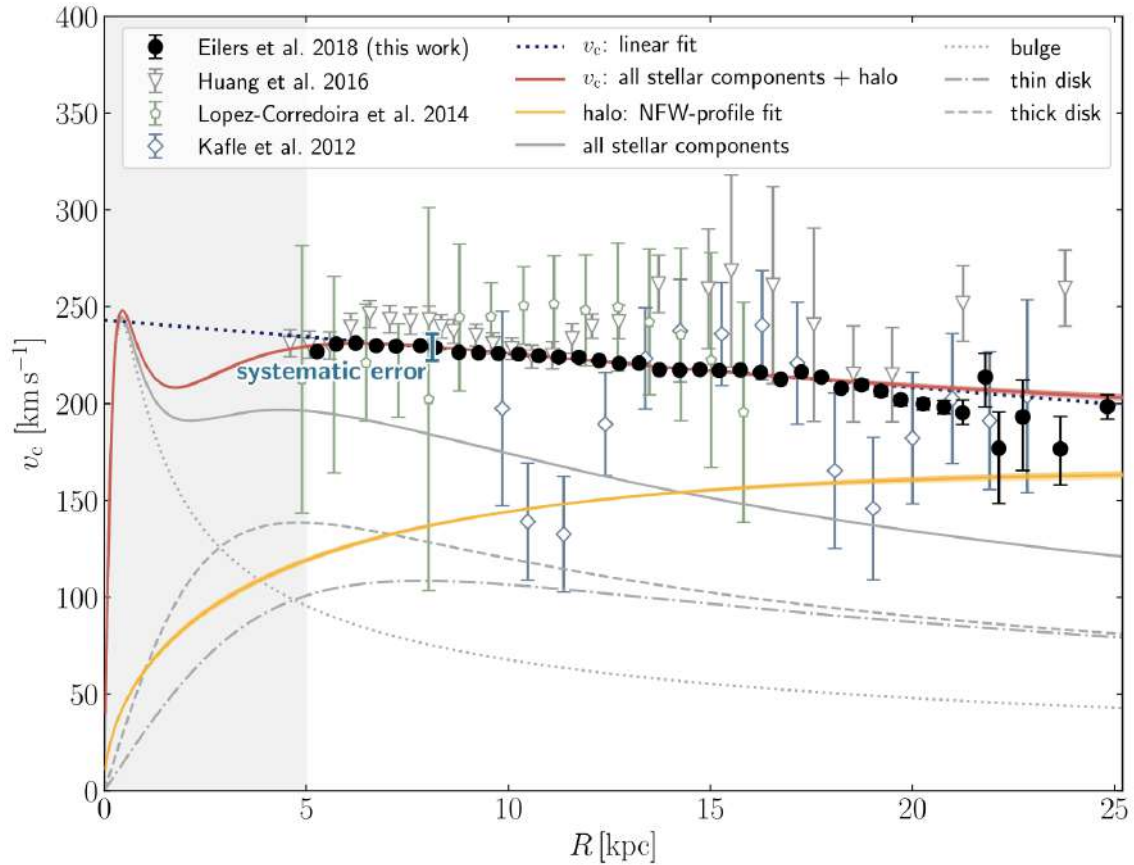
FIGURE 12.15 – Courbe de rotation Galactique. Le trait gris représente la courbe correspondant aux seules composantes visibles, qui ne reproduit pas les observations. La courbe jaune correspond à un modèle de halo de matière noire (profil de Navarro-Frenk-White [113]) et la courbe rouge correspond à la somme des composantes stellaires et du halo de matière noire. Figure issue de [114].
