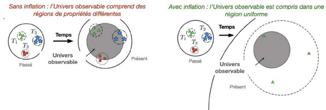
FIGURE 14.17 – Le paradigme de l'inflation. Figure adaptée d'un schéma de N. Strobel.
