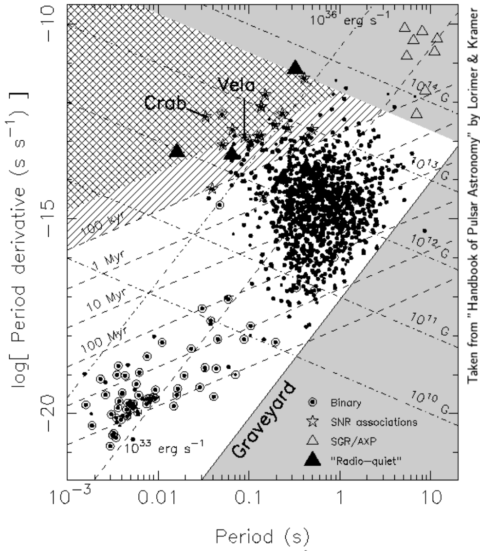
FIGURE 8.5 – Diagramme période-dérive des pulsars.
