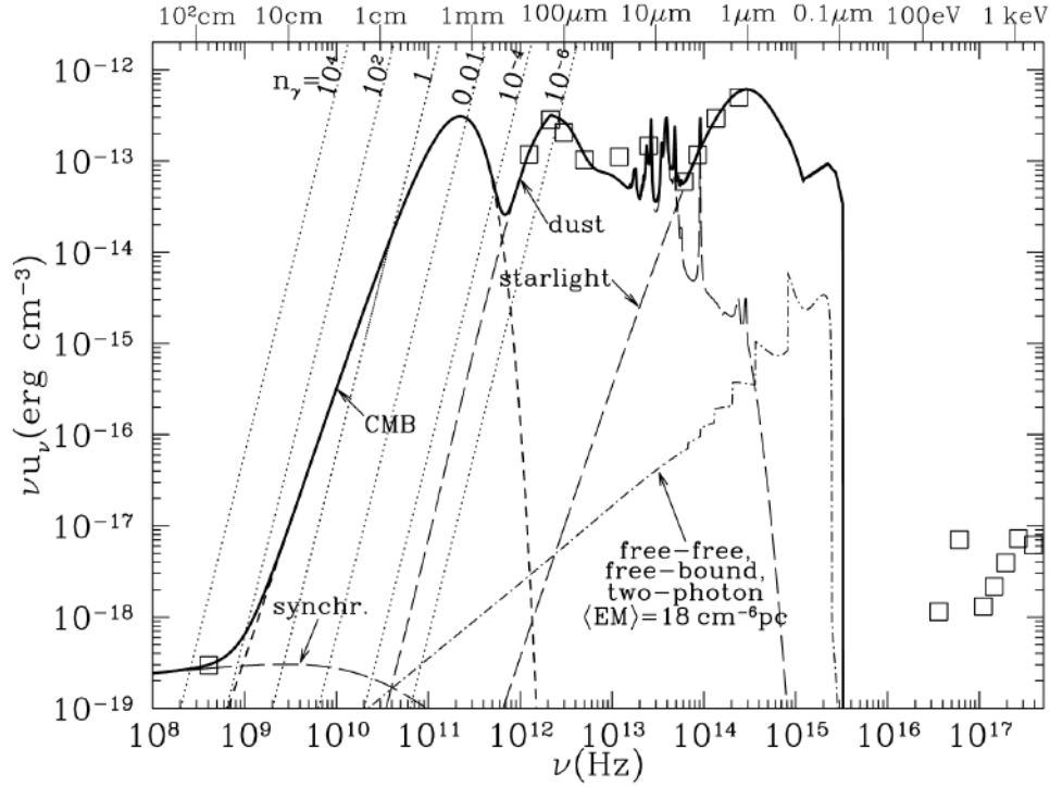
FIGURE 1.7 – Le champ de rayonnement interstellaire standard , montrant les différentes sources de rayonnement (synchrotron Galactique, fond diffus cosmologique, émission thermique des poussières, rayonnement stellaire, rayonnement de freinage et continua de recombinaison, ...). Figure issue de [3].
