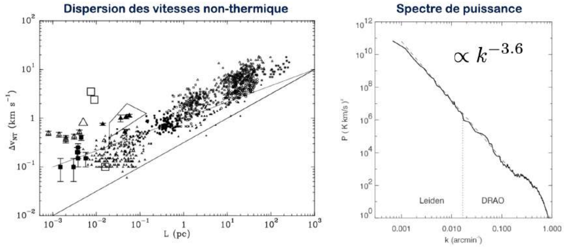
FIGURE 10.32 – Signatures observationnelles de la turbulence. Dispersion des vitesses nonthermique en fonction de l'échelle [69] (à gauche) et spectre de puissance de l'émission HI dans Ursa Major [70] (à droite).
