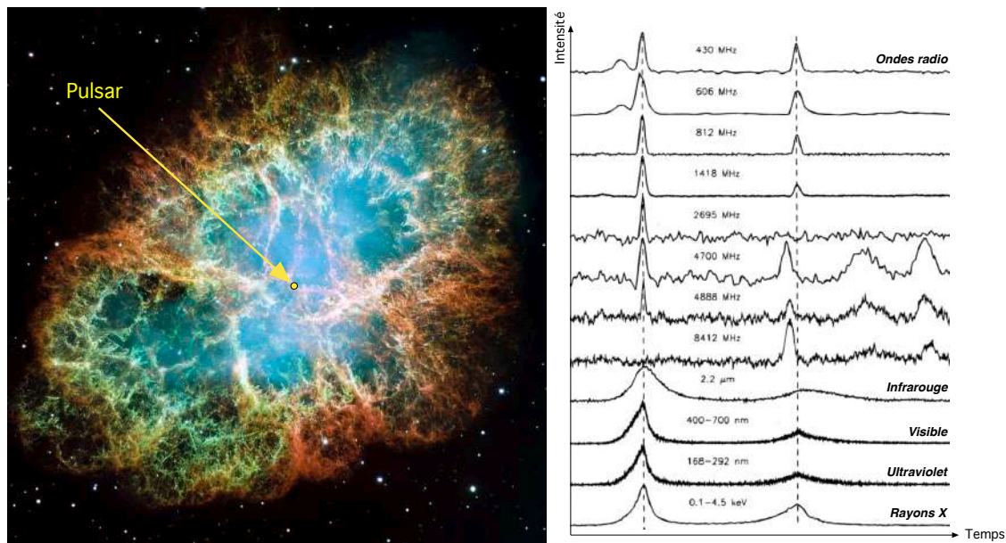
FIGURE 6.3 – Phénomène de pulsar. Sur l'image de gauche, la nébuleuse du Crabe observée en optique par le télescope spatial Hubble (Crédit : NASA/STScI). Les "pulses" d'émission issus du pulsar qui se trouve au centre de la nébuleuse sont représentés en fonction du temps sur les courbes à droite, pour différentes fréquences, des ondes radio en haut aux rayons X en bas. La durée totale représentée sur chaque courbe correspond à une période unique de rotation du pulsar, à savoir 33,736 ms. (Figure adaptée de D. A. Moffett & T. H. Hankins, The Astrophysical Journal , 468, 779, 1996 [ https://arxiv.org/abs/astro-ph/9604163 ]).
