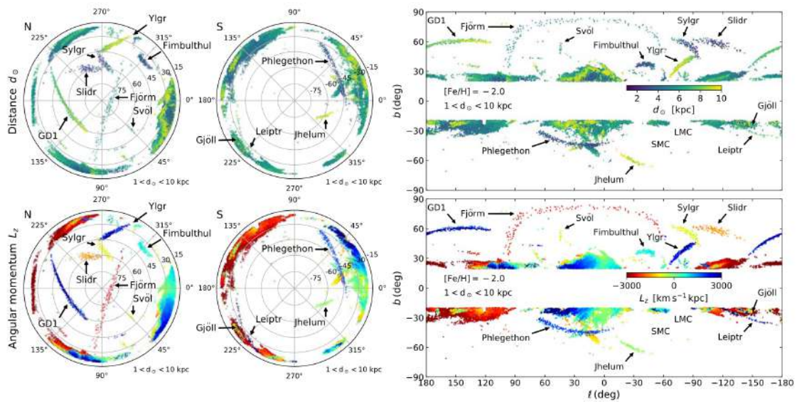
FIGURE 12.9 – Courants stellaires dans le halo Galactique. Figure issue de [101].
