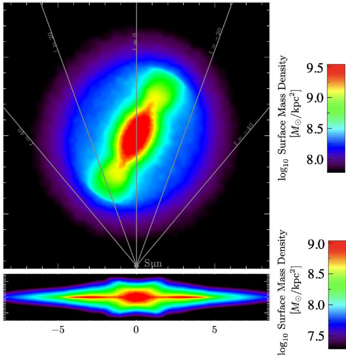
FIGURE 12.14 – Simulation numérique du bulbe et de la barre Galactiques. Figure issue de [112].
