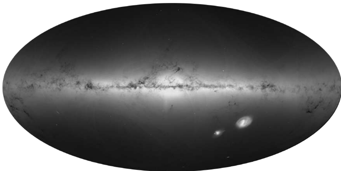
FIGURE 12.1 – Distribution dans le ciel de 1.7 milliards de sources observées par Gaia.
