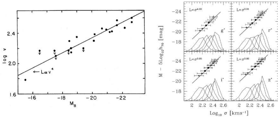
FIGURE 13.17 – Relation de Faber-Jackson. Le panneau de gauche présente la corrélation dans l'article original [138] et celui de droite montre des corrélations obtenues sur un ensemble beaucoup plus important (9000) de galaxies elliptiques dans différentes bandes [139].
