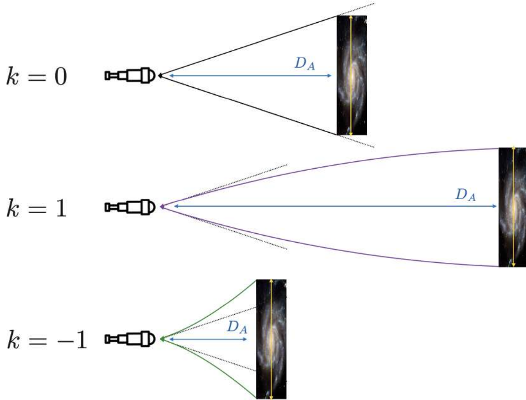
FIGURE 14.8 – Distance angulaire. Une galaxie de même taille physique apparaissant avec une même taille angulaire peut être à des distances différentes en fonction de la courbure de l'espace.
