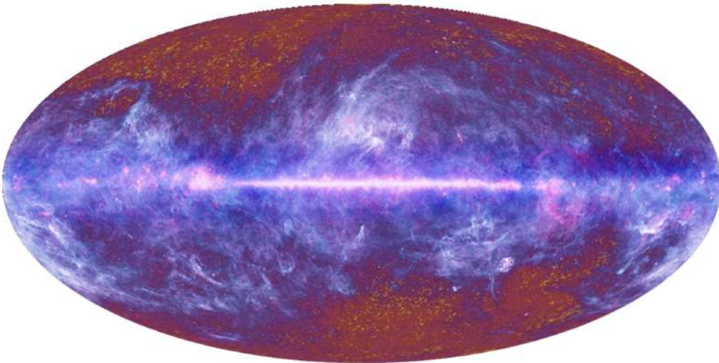
FIGURE 10.27 – Emission FIR de la poussière Galactique observée par Planck [60].
