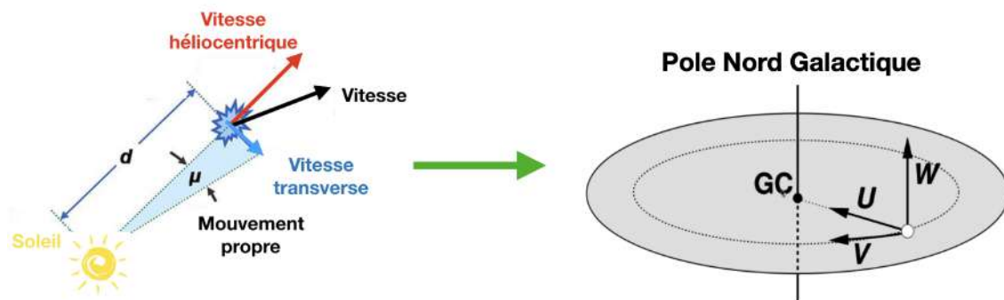
FIGURE 12.4 – Détermination de la cinématique des étoiles.
