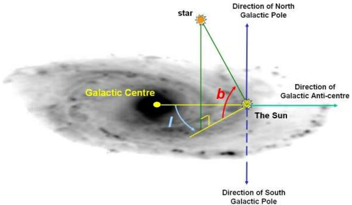
FIGURE 12.3 – Les coordonnées Galactiques
