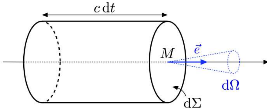
FIGURE 2.1 – Définition de l'intensité spécifique dans la direction normale. Notations utilisées pour définir l'intensité spécifique dans la direction \vec{e} normale à l'élément de surface.
