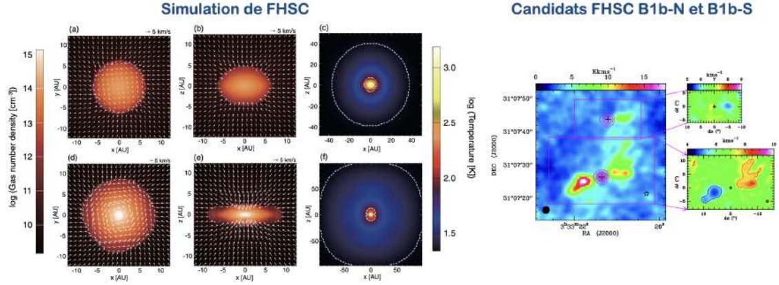
FIGURE 11.26 – Premiers cœurs hydrostatiques. Simulations (à gauche) [88] et observations d'objets candidats (à droite) [89].
