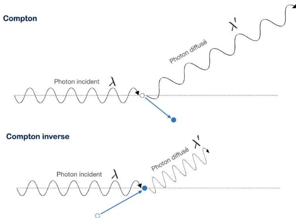
FIGURE 2.13 – Diffusion Compton et Compton inverse.
