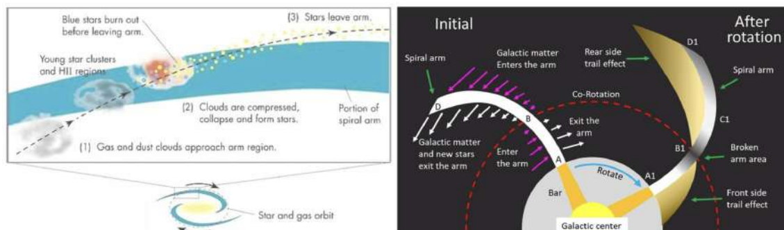
FIGURE 13.9 – Bras spiraux et formation stellaire. Le panneau de gauche schématise l'impact du passage d'une onde de densité sur un nuage de gaz et de poussières ( https://universe-review.ca/F05-galaxy08.htm ) et celui de droite représente la structure d'un bras et montre le rayon de corotation.
