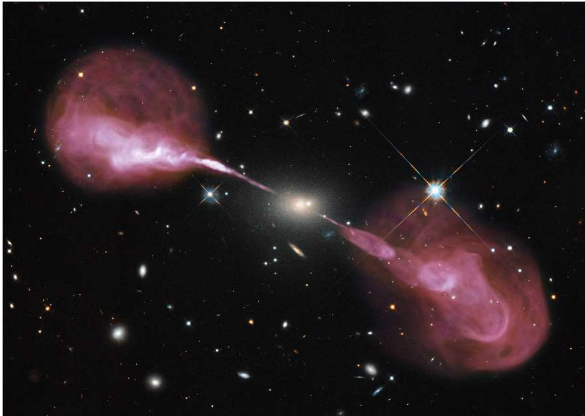
FIGURE 13.25 – La galaxie active Hercules A. À l'image en optique obtenue avec HST est superposée l'observation de lobes radio avec le VLA.
