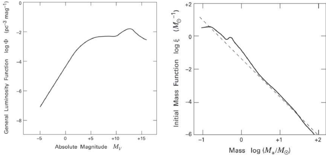
FIGURE 11.13 – Fonctions de luminosité et de masse initiale. Fonction de luminosité (à gauche) et fonction de masse initiale dans le voisinage solaire (à droite). Figures issues de [25].
