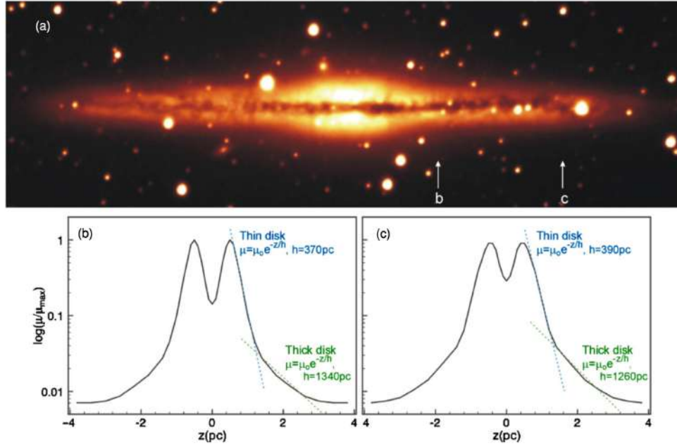
FIGURE 12.6 – Disques épais et minces dans NGC891. Les courbes du bas sont des coupes de l'image du haut aux deux positions b et c , perpendiculairement au disque. On y voit les deux composantes, mince et épaisse, et l'effet de l'absorption par les poussières dans le plan moyen. Figures issues de [98].
