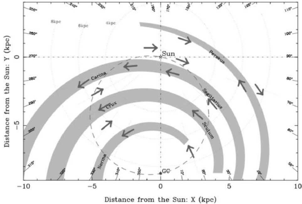
FIGURE 10.31 – Structure du champ magnétique Galactique [67].
