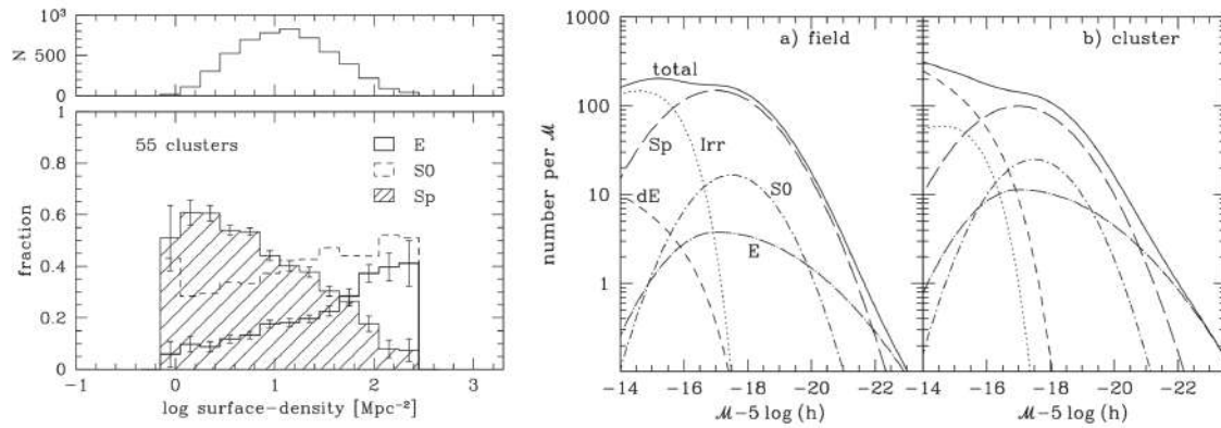
FIGURE 13.28 – Statistiques des galaxies d'amas et du champ. Le panneau de gauche montre les histogrammes des elliptiques (E), lenticulaires (S0) et spirales (Sp) en fonction de la densité d'objets. Les galaxies dans les amas sont donc à droite de la répartition et celle du champ à gauche. Le panneau de droite montre les fonctions de luminosité des différents types de galaxies dans le champ (sous-panneau a) et dans les amas (sous-panneau b).
