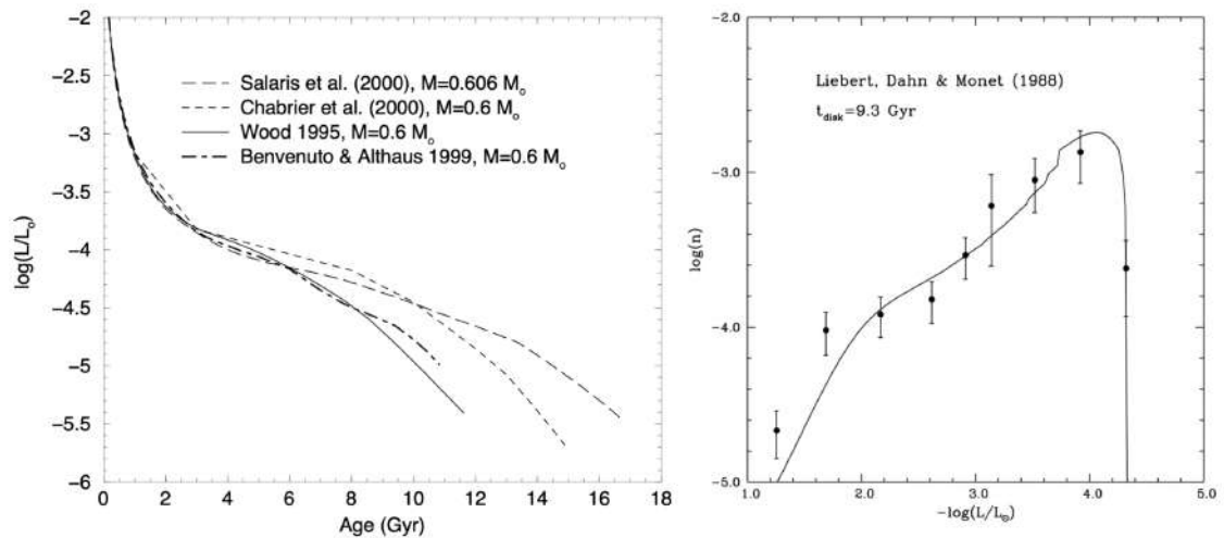
FIGURE 7.8 – Refroidissement des naines blanches. La figure de gauche montre la luminosité d'une naine blanche en fonction du temps, pour différents modèles de refroidissement (Figure issue de [41]). La figure de droite montre la fonction de luminosité des naines blanches, avec une coupure à basse luminosité correspondant à l'âge du disque de la Galaxie (Figure issue de [42]).
