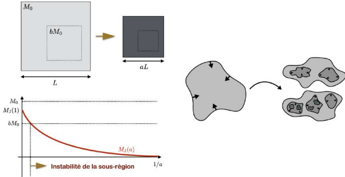
FIGURE 11.24 – Fragmentation hiérarchique. Modèle schématique (à gauche) et représentation plus "réaliste" de son effet sur un nuage en effondrement (à droite).
