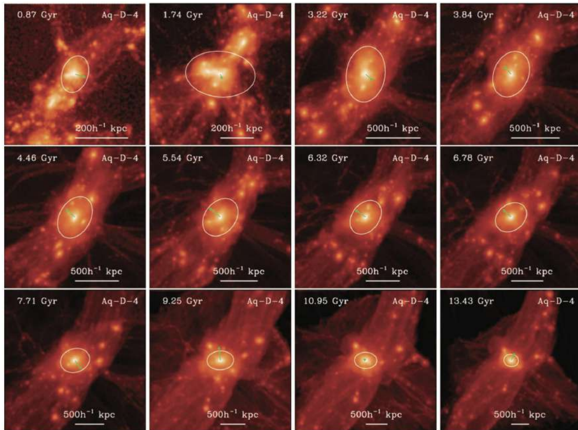
FIGURE 12.17 – Simulation numérique de l'évolution d'un halo de matière noire. Les différents panneaux correspondent à différentes époques d'une même structure dans une simulation N corps et indiquent la forme du halo de matière noire (contour blanc) et l'orientation de son petit axe (flèche verte). Figure issue de [117].
