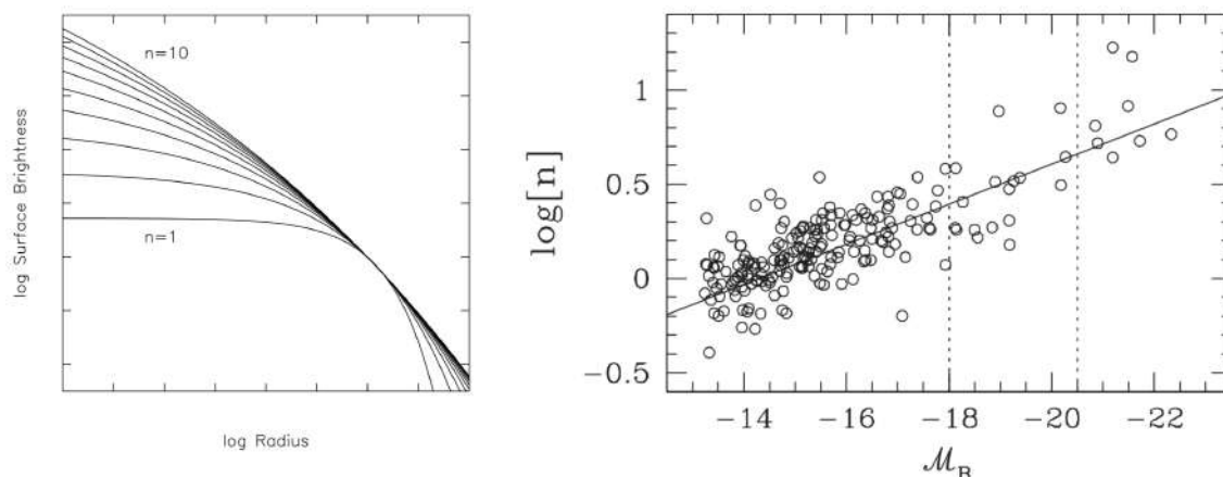
FIGURE 13.15 – Profils de Sérsic. Le panneau de gauche montre différents profils pour n = 1 à n = 10 et celui de droite montre la corrélation de n avec la magnitude de la galaxie.
