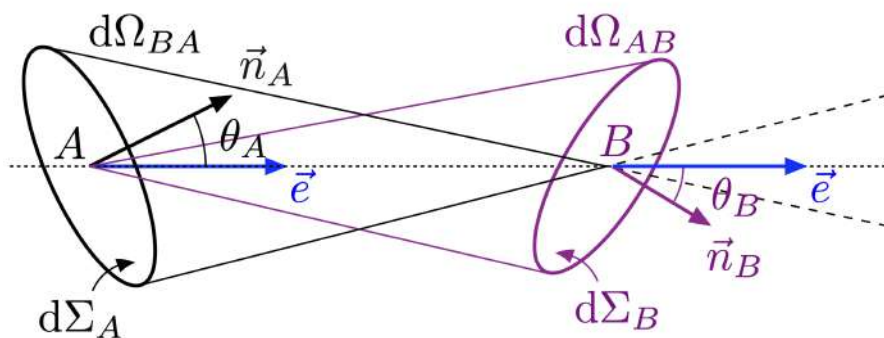
FIGURE 2.4 – Conservation de I_\nu dans le vide. Notations utilisées pour établir la conservation de l'intensité spécifique entre les points A et B lorsqu'aucune interaction n'intervient le long du trajet AB entre les deux points.
