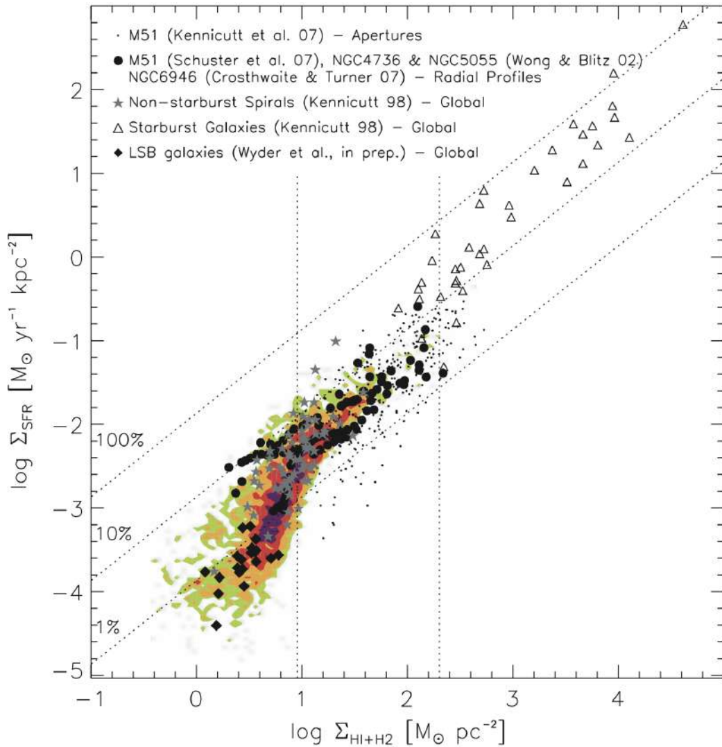
FIGURE 10.2 – Relation de Schmidt-Kennicutt composite, issue de [46]. Les droites en pointillés indiquent les taux de formation stellaires ( \Sigma_{\text{SFR}} ) nécessaires pour convertir 1%, 10% et 100% d'une masse de gaz donnée ( \Sigma_{\text{H}} = \Sigma_{\text{HI}+\text{H}_2} ) en étoiles sur un temps de 10^8 ans, à SFR constant.
