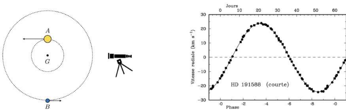
FIGURE 5.10 – Exemple de binaire spectroscopique. Le schéma de gauche montre le principe de la détection, la figure de droite montre la vitesse radiale en fonction du temps pour l’étoile HD191588 [30].
