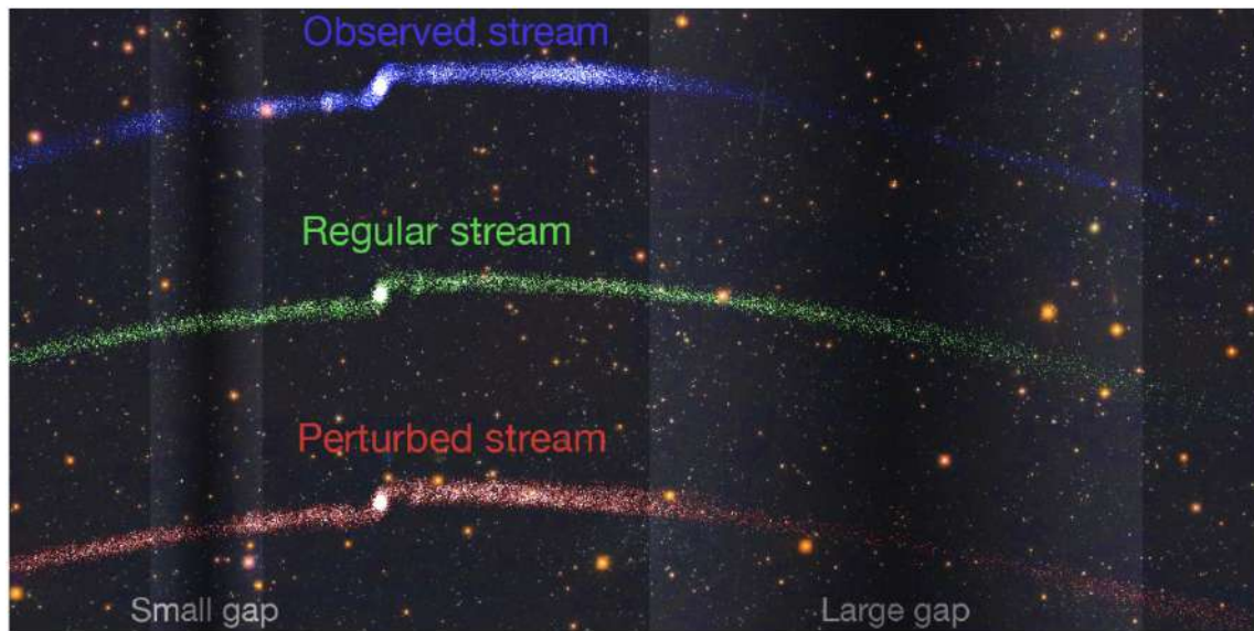
FIGURE 12.18 – Effet d'un sous-halo sur un courant stellaire. Le courant Palomar 5 observé est représenté en bleu. Les courants vert et rouge sont des simulations de Palomar 5 sans perturbation par un sous-halo (en vert) et avec une perturbation (en rouge). Crédit : V. Belokurov, D. Erkal, S.E. Koposov (IoA, Cambridge).
