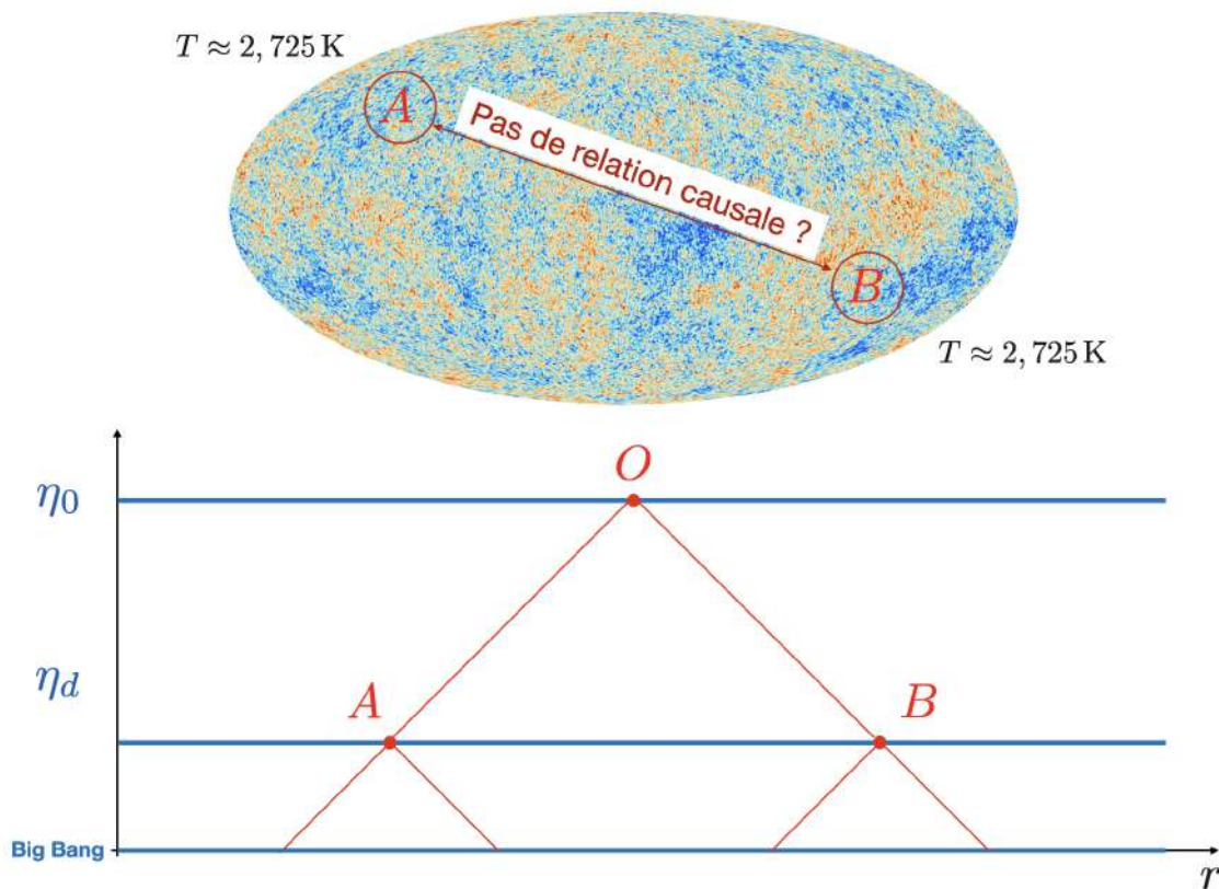
FIGURE 14.16 – Le problème de l'horizon. Les conditions physiques aux points A et B sur la surface de dernière diffusion sont déterminées par leur histoire, incluse dans leurs cônes de lumière depuis le Big Bang, qui ne se recouvrent pas et ne peuvent donc imposer l'homogénéité en A et B . Figure adaptée de [2].
