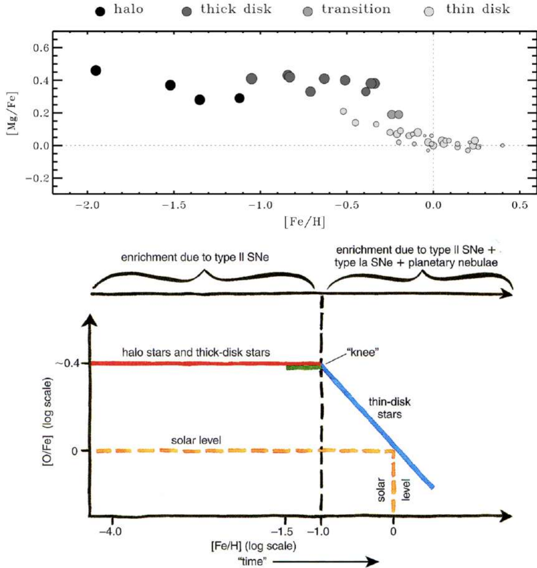
FIGURE 12.19 – Plan d'abondances [Mg/Fe] - [Fe/H] . Le panneau du haut montre ces abondances pour des étoiles du voisinage solaire, dans les différentes structures du disque et du halo [119], le panneau du bas présente l'interprétation schématique de ces tendances [120].
