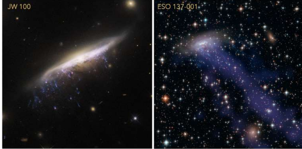
FIGURE 13.27 – Exemples de galaxies "méduses".
