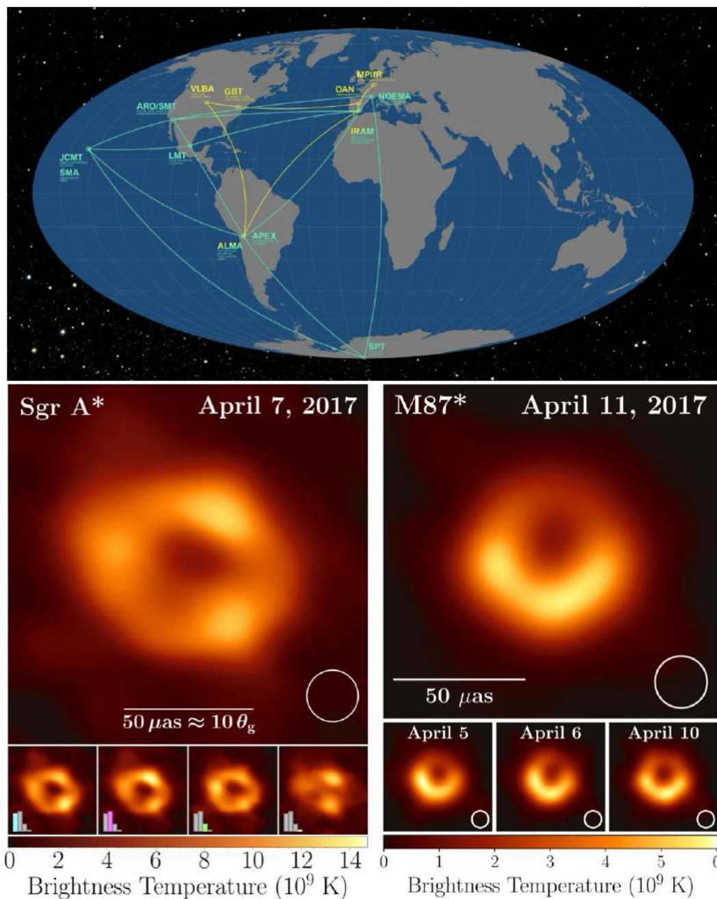
FIGURE 1.24 – VLBI avec l'Event Horizon Telescope (EHT) . Positions des antennes formant le réseau EHT (en haut, Wikimedia Commons ) et premières images directes de trous noirs supermassifs au centre de notre Galaxie (en bas à gauche) [11] et au centre de la galaxie M87 (en bas à droite) [12].
