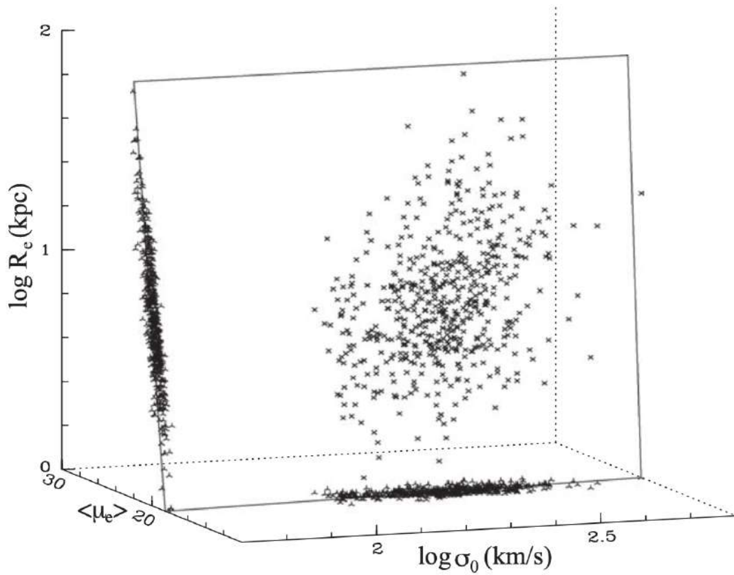
FIGURE 13.16 – Plan fondamental des galaxies elliptiques.
