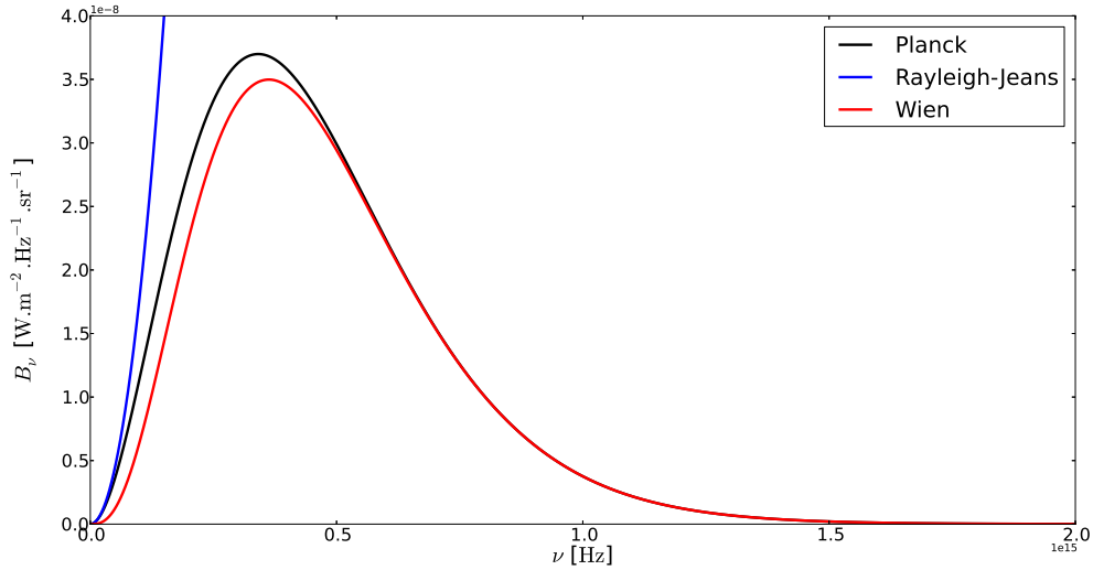
FIGURE 3.6 – Lois de Planck, Rayleigh-Jean et Wien. Loi de Planck (en noir), loi de Rayleigh-Jeans (en bleu) et loi de Wien (en rouge), pour un corps noir à T = 5800 \text{ K} .
