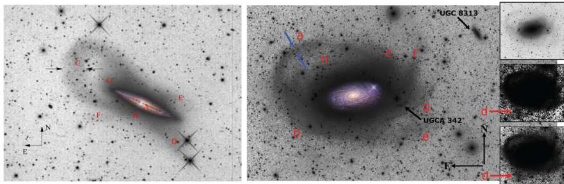
FIGURE 12.10 – Halos stellaires de galaxies externes. Le panneau de gauche montre le cas de NGC 4013 [102] et celui de droite le cas de M63 [103].
