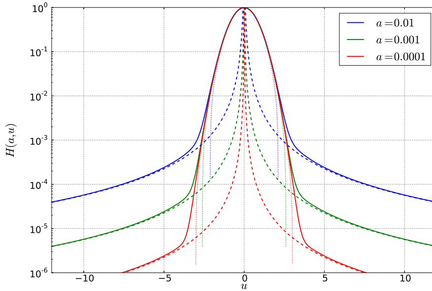
FIGURE 4.4 – Profils de Voigt . On montre en traits pleins les cas a = 10^{-2} (bleu), a = 10^{-3} (vert) et a = 10^{-4} (rouge). Les courbes en pointillés représentent les approximations Gaussiennes au centre de chaque profil, et les courbes en tirets les approximations Lorentziennes dans les ailes. Noter que l'axe des ordonnées est en échelle logarithmique.
