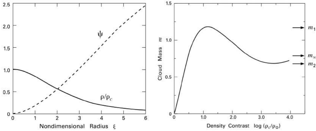
FIGURE 11.19 – Equation de Lane-Emden isotherme. Solution (à gauche) et évolution de la masse (adimensionnée) en fonction du contraste de densité pour un nuage borné par la pression extérieure (à droite). Figures issue de [25].
