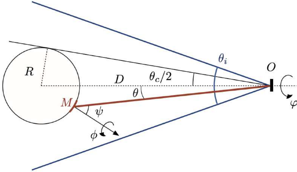
FIGURE 2.5 – Décroissance du flux en raison du carré inverse de la distance.
