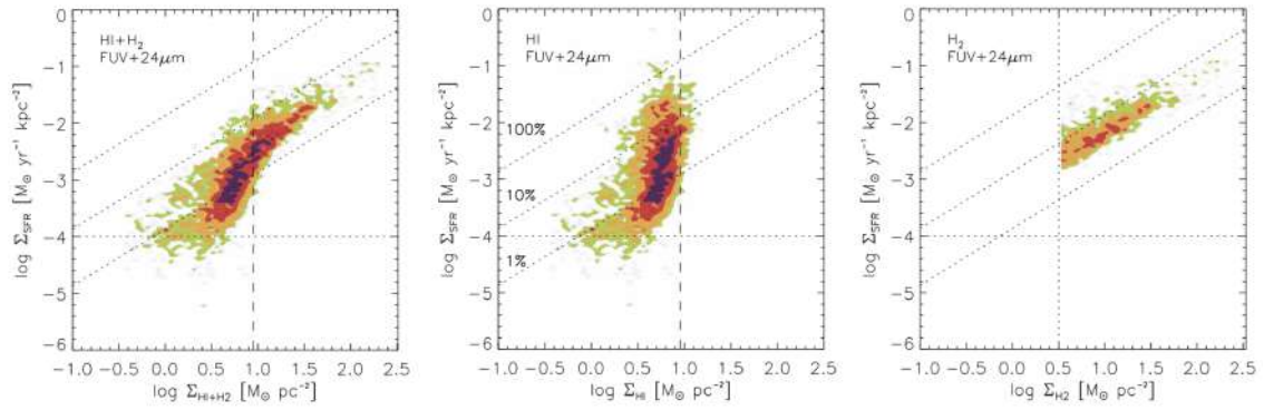
FIGURE 13.22 – Relation de Kennicutt-Schmidt pour un ensemble de galaxies spirales proches Figure issue de [46].
