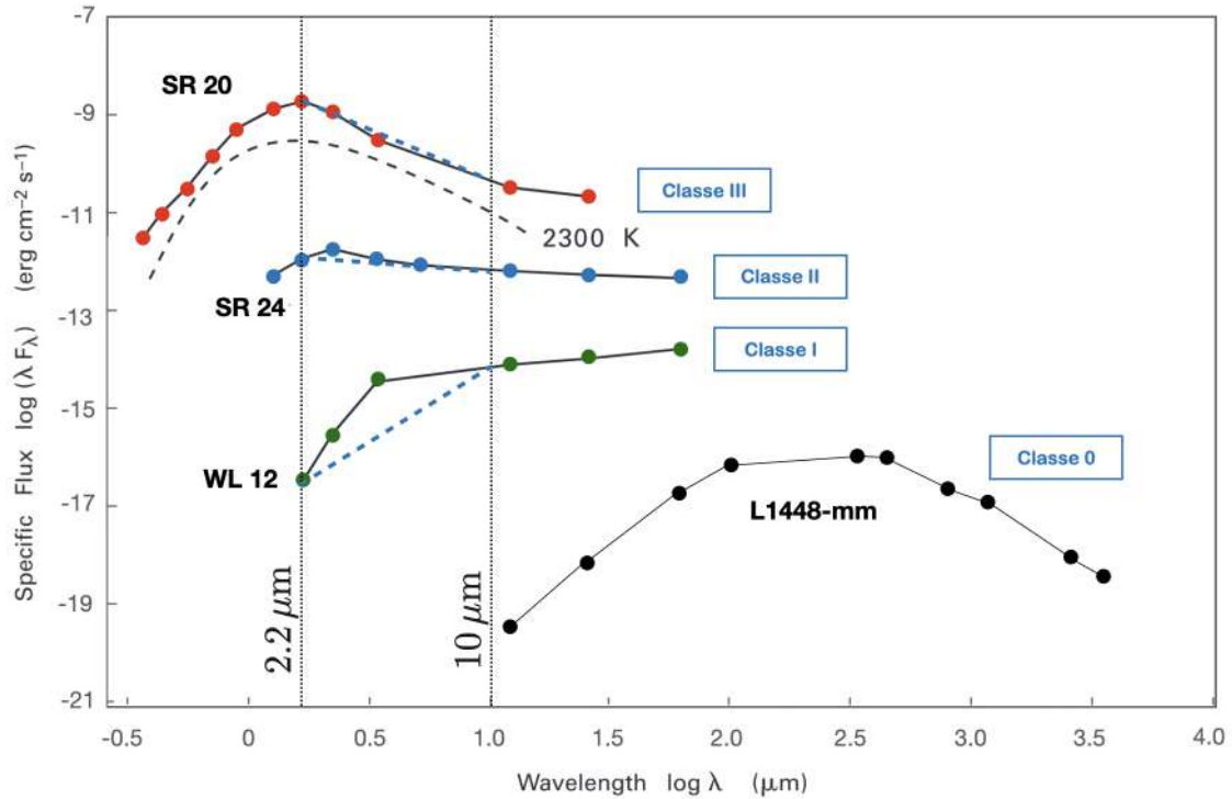
FIGURE 11.5 – Spectres corrigés du rougissement interstellaire pour différents objets stellaires jeunes (classes 0 à III). Le spectre d'un corps noir à 2300 K est aussi indiqué. Figure adaptée de [25].
