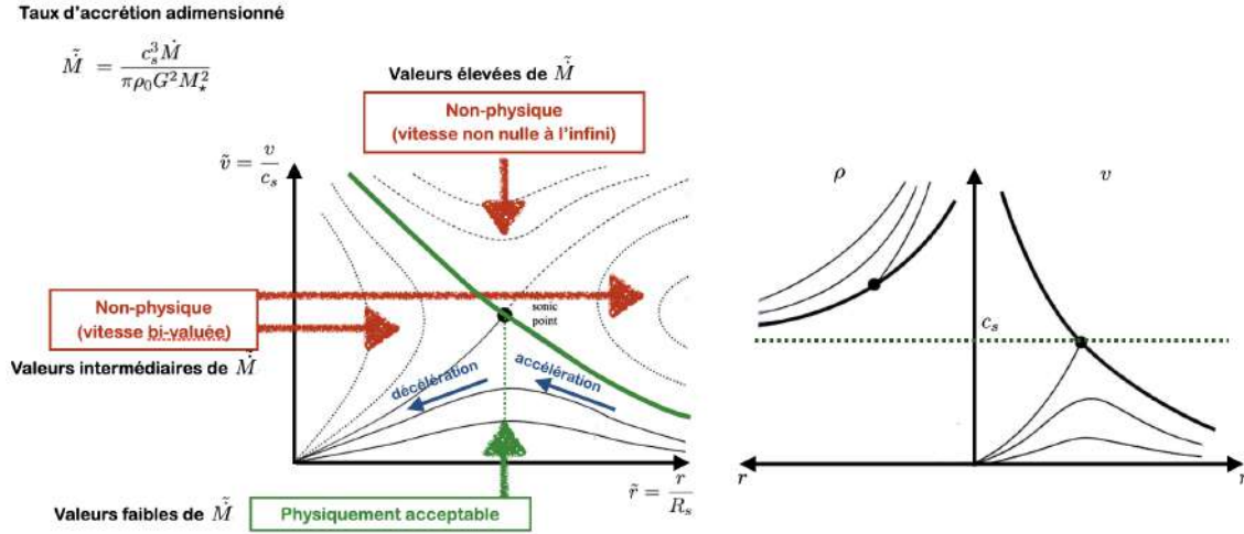
FIGURE 11.28 – Solutions de l'accrétion de Bondi. Solutions \tilde{v}(\tilde{r}) pour différents taux d'accrétions adimensionnés \tilde{M} (à gauche) et profils de vitesse et de densité pour les solutions physiquement acceptables (à droite). Figure adaptée de [80].
