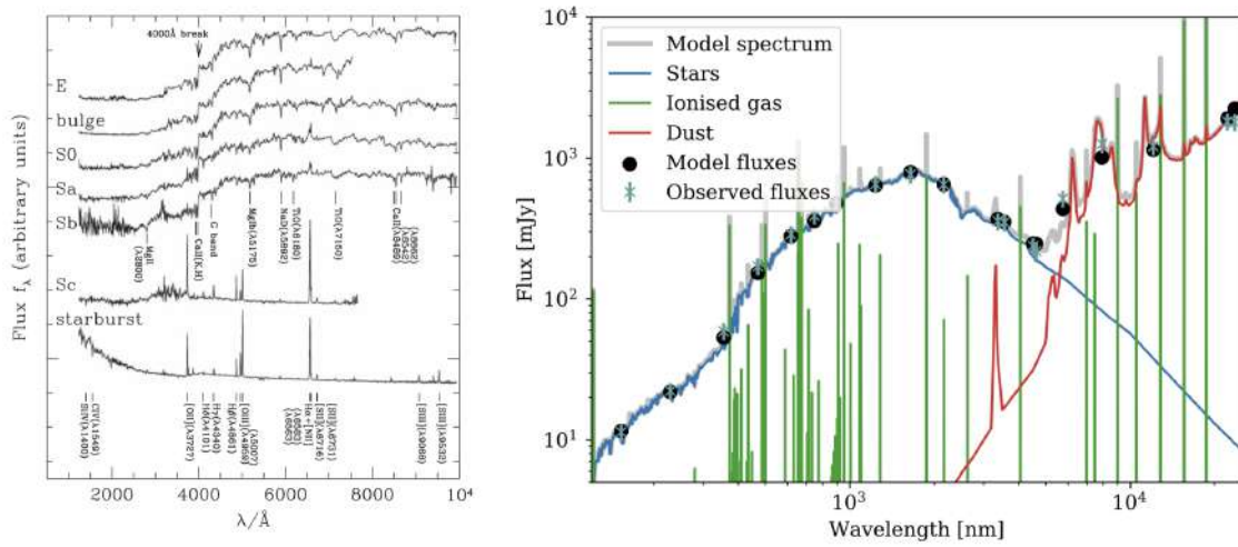
FIGURE 13.5 – Différents spectres de galaxies. Le panneau de gauche montre des spectres pour différents types de galaxies (figure issue de [131]) et celui de droite montre l'ajustement du spectre de la galaxie spirale NGC 4321 par le biais du code CIGALE (figure issue de [130]).
