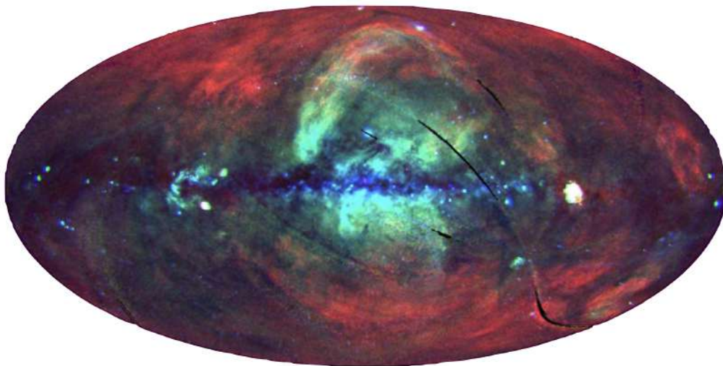
FIGURE 10.30 – Relevé ROSAT dans les rayons X mous. (rouge : 0.2-0.4 keV, vert : 0.5-0.9 keV, bleu : 0.9-2.0 keV) [66].
