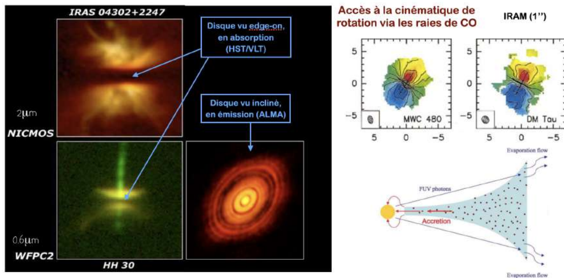
FIGURE 11.31 – Disques protoplanétaires. Observations en absorption et en émission (à gauche), cartes de rotation obtenues à partir des raies de CO (en haut à droite), et schéma de la structure évasé d'un disque (en bas à droite).
