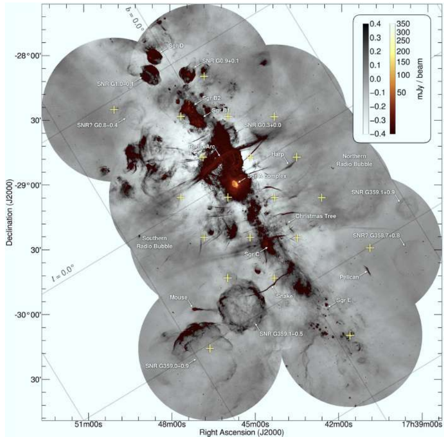
FIGURE 6.7 – Le centre Galactique. Image obtenue en radio par l'interféromètre MeerKAT. Le trou noir central se trouve dans la région "Sgr A complex". Figure issue de [37].
