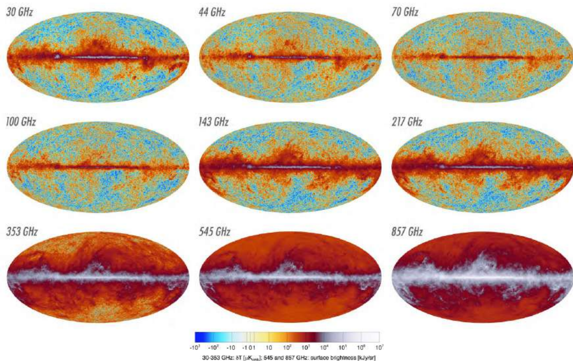
FIGURE 1.6 – Le ciel vu par Planck dans ses neuf bandes de fréquences. Les trois fréquences les plus basses (30 à 70 GHz) correspondent à l'instrument basses fréquences (LFI) et les six autres (100 à 857 GHz) à l'instrument hautes fréquences (HFI). Figure issue de [2]
