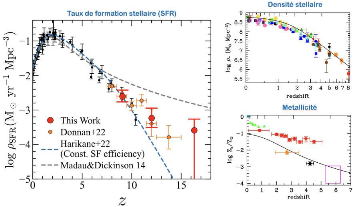
FIGURE 10.7 – Evolution du taux de formation stellaire (à gauche), de la densité des étoiles (en haut à droite) et de la métallicité (en bas à droite) avec le redshift. Les figures de droite sont issues de [51], la figure de gauche est plus récente, incluant des mesures avec JWST, et est issue de [52].
