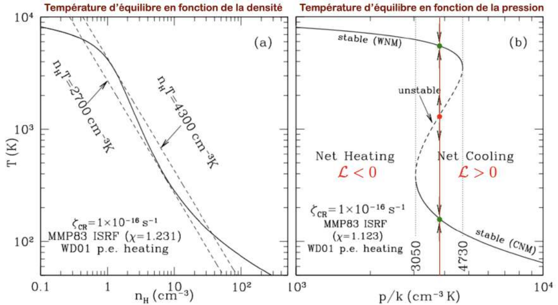
FIGURE 10.15 – Température d'équilibre du H I . Elle est représentée en fonction de la densité du gaz (à gauche) et de la pression (à droite). Figure adaptée de [3].
