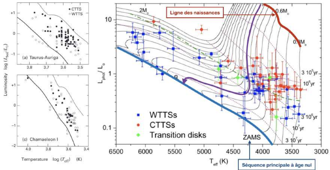
FIGURE 11.9 – ZAMS et ligne des naissances. À gauche : diagrammes de Hertzsprung-Russell d'associations T dans Taurus et Chamaeleon, montrant les T Tauri classiques et à raies faibles, la ligne des naissance et la ZAMS. Figure issue de [25]. À droite, sur le cas d'une autre association, on montre les trajectoires d'évolution d'étoiles de différentes masses. Figure adaptée de [74].
