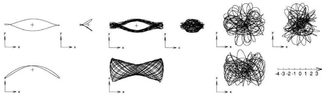
FIGURE 12.13 – Orbites stellaires formant un bulbe en forme de "cacahouète". Les orbites représentées sont périodiques (à gauche), quasi-périodiques (au milieu) ou chaotiques (à droite). Figure issue de [110].
