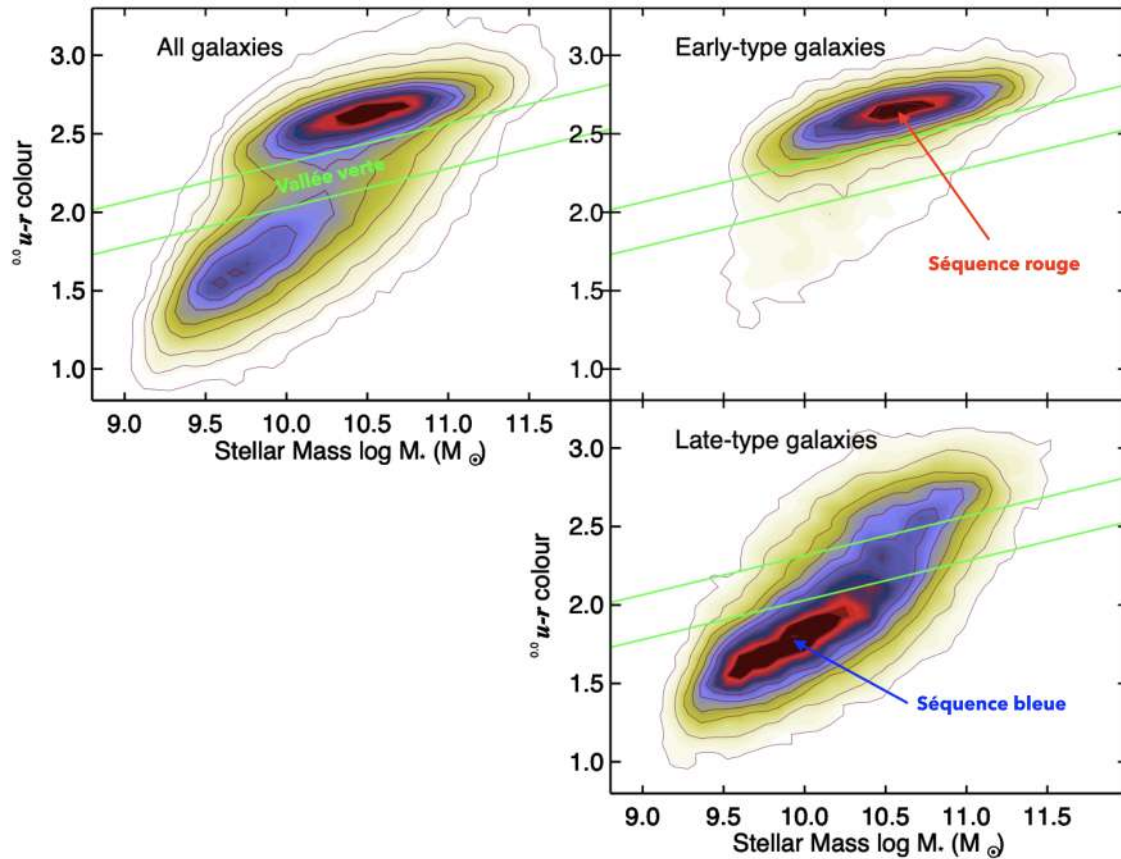
FIGURE 13.3 – Séquences rouge et bleue, vallée verte. Figure adaptée de [129].
