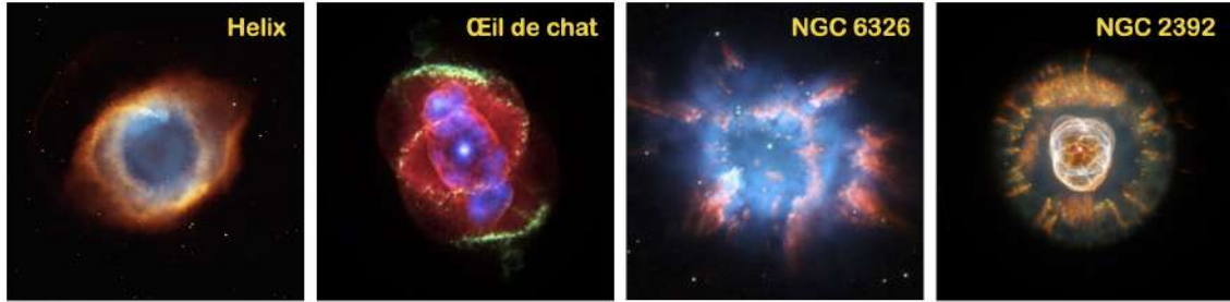
FIGURE 10.13 – Quelques nébuleuses planétaires.
