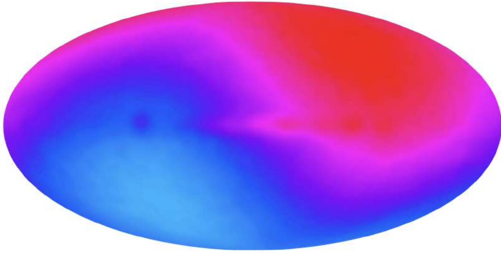
FIGURE 14.13 – Emission du corps noir cosmologique (CMB) montrant l'effet de dipôle. L'échelle des couleurs va de -2.5 \text{ mK} (bleu) à +3.5 \text{ mK} (rouge) autour de la valeur moyenne de l'émission du CMB. Crédit : DMR/COBE/NASA.
