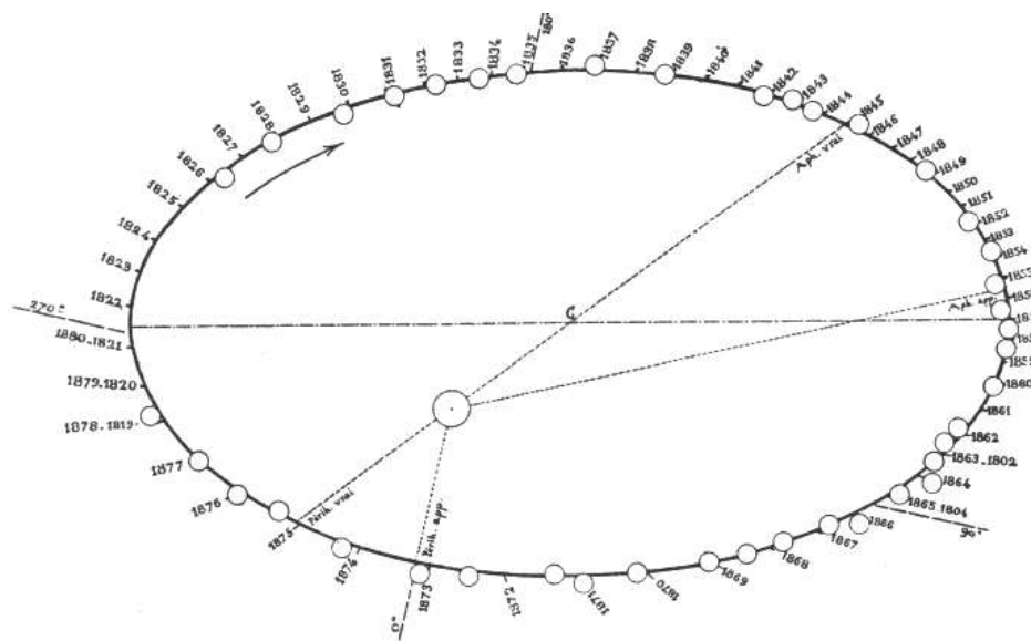
Fig. 7/3. — Orbite apparente de l'étoile double ξ Grande Ourse.
