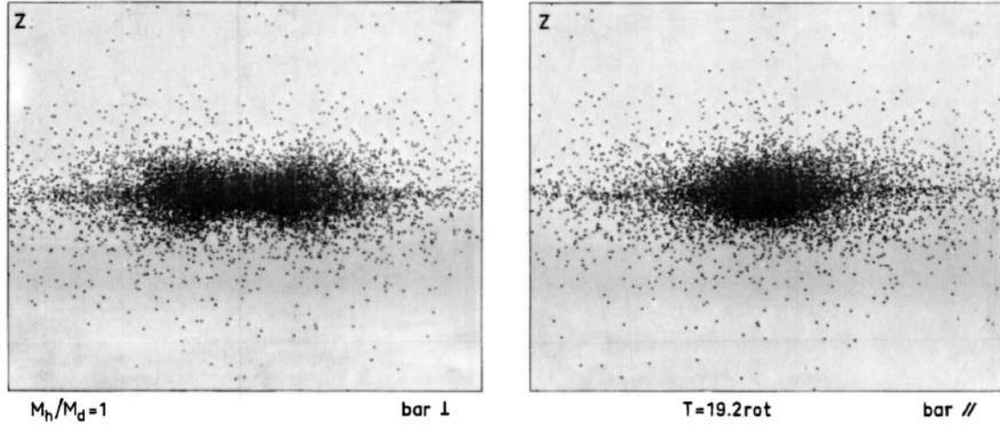
FIGURE 13.10 – Morphologie d'un bulbe central. Les figures montrent des vues de simulations d'une barre, perpendiculairement à celle-ci à gauche et parallèlement à droite. Figure issue de [111].
