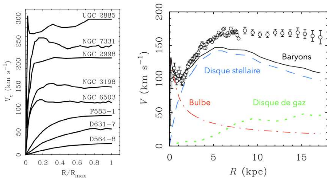
FIGURE 13.12 – Courbes de rotation de galaxies spirales. Le panneau de gauche montre des courbes de rotation de différentes galaxies, celui de droite montre les contributions de différentes composantes visibles à la courbe de rotation d'une galaxie (NGC 6946). Figure adaptée de [133].
