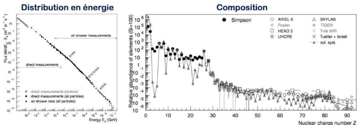
FIGURE 10.24 – Distribution en énergie et composition des rayons cosmiques. Figures issues de [3].
