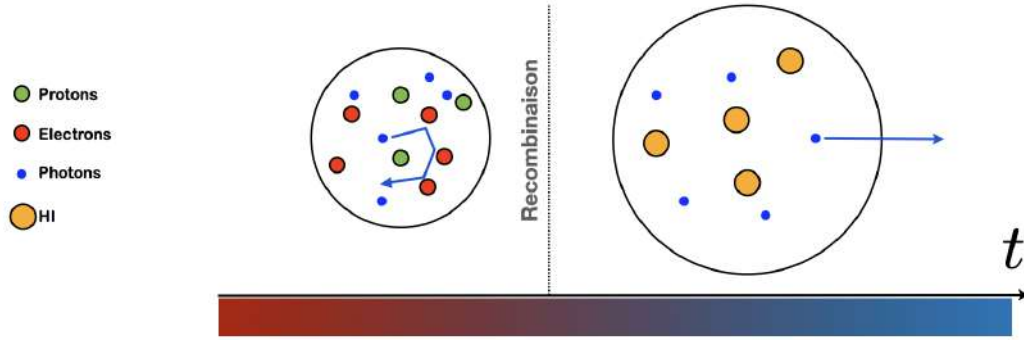
FIGURE 14.11 – La recombinaison.
