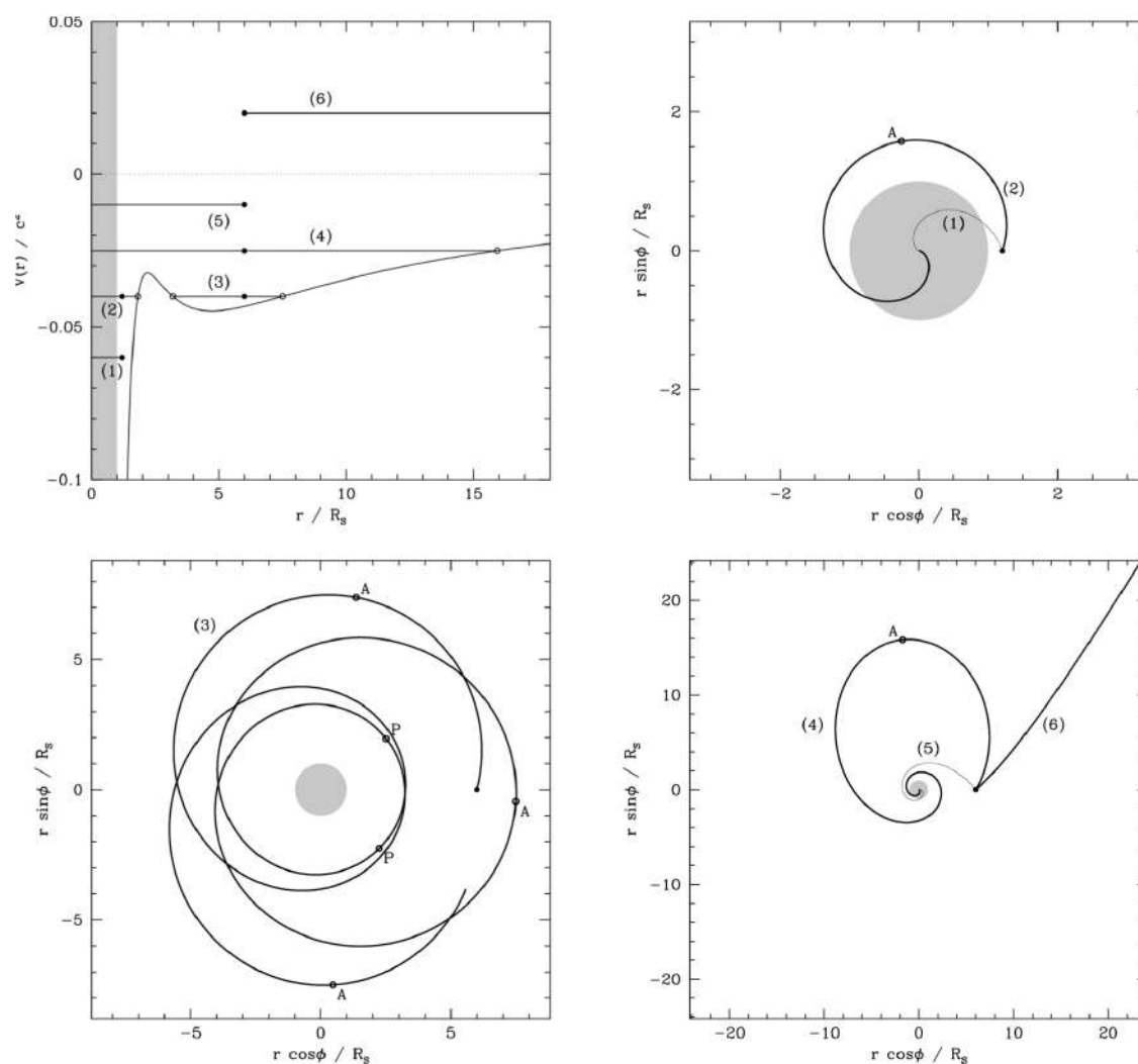
FIGURE 9.4 – Trajectoires autour d'un trou noir de Schwarzschild. La figure en haut à gauche montre le potentiel effectif V (noté ici V/c^2 ) en fonction du rayon normalisé r/R_S . La région interne à l'horizon est présentée en grisé, et six exemples de trajectoires issues de (r = r_0, \phi = 0) , notées (1) à (6). Les traits horizontaux traduisent la conservation de l'énergie, les points noirs le rayon initial r_0 et les cercles les passages éventuels à l'apoastre ou au périastre. Les trois autres figures représentent les trajectoires correspondantes. [Crédit : F. Daigne]
