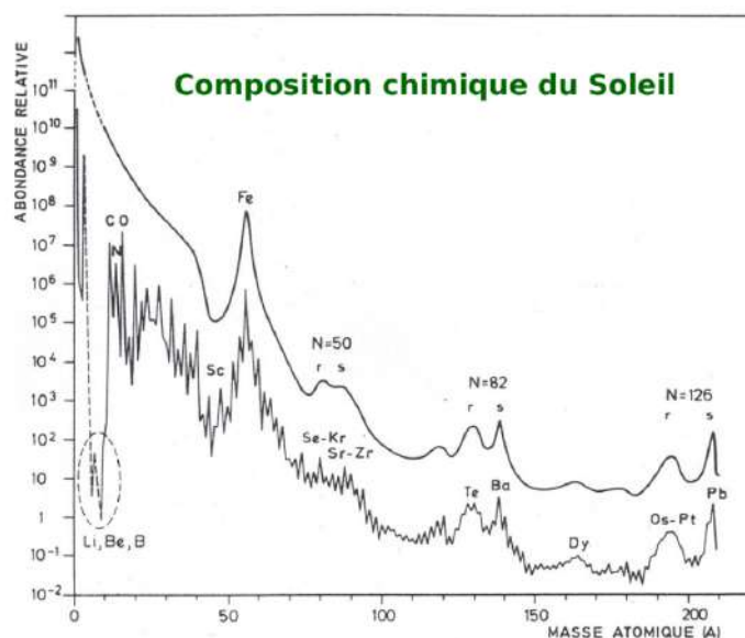
FIGURE 5.4 – Composition chimique du Soleil. Les chiffres de la table de droite sont les abondances en nombre d'atomes et non les fractions de masse [28].
