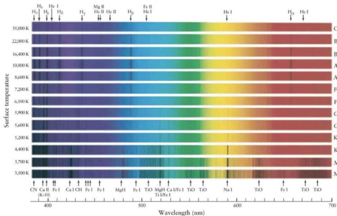
FIGURE 5.6 – Spectres stellaires. Pour chaque type spectral (à droite), on indique la température effective (à gauche) et les raies d'absorption principales (en haut et en bas).
