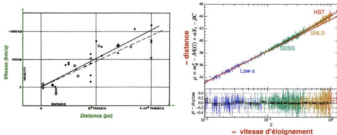
FIGURE 14.2 – La loi de Hubble-Lemaître . La figure de gauche est issue de l'article original de Hubble [146], celle de droite montre des mesures sur une plus grande plage de redshifts et souligne la déviation à la loi linéaire, correspondant à l'accélération de l'expansion [147].
