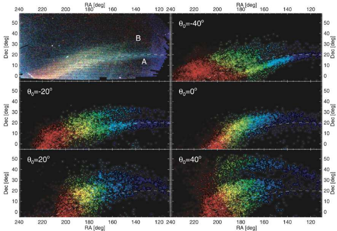
FIGURE 12.8 – Le courant du Sagittaire. Le panneau en haut à gauche montre la distribution stellaire du courant du Sagittaire, les couleurs codant différentes distances héliocentriques. Les autres panneaux montrent des résultats de simulations numériques, pour différentes inclinaisons du disque de la galaxie naine par rapport à son plan orbital. Figure issue de [100].
