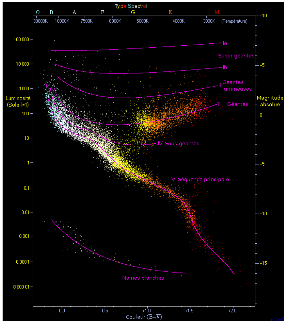
FIGURE 5.7 – Diagramme de Hertzsprung-Russell. Les classes de luminosité sont indiquées, des super-géantes aux naines blanches. Les sous-naines n'apparaissent pas dans ce diagramme particulier. [Crédit : R. Powell / Wikimedia Commons.]
