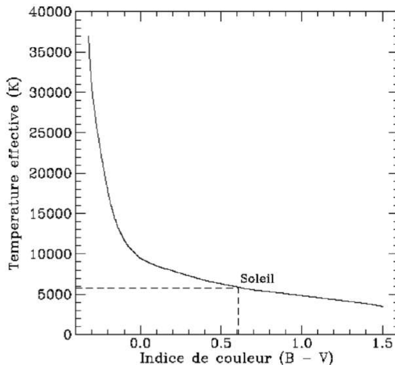
FIGURE 5.3 – Relation indice de couleur - température effective. Données issues de [27].
