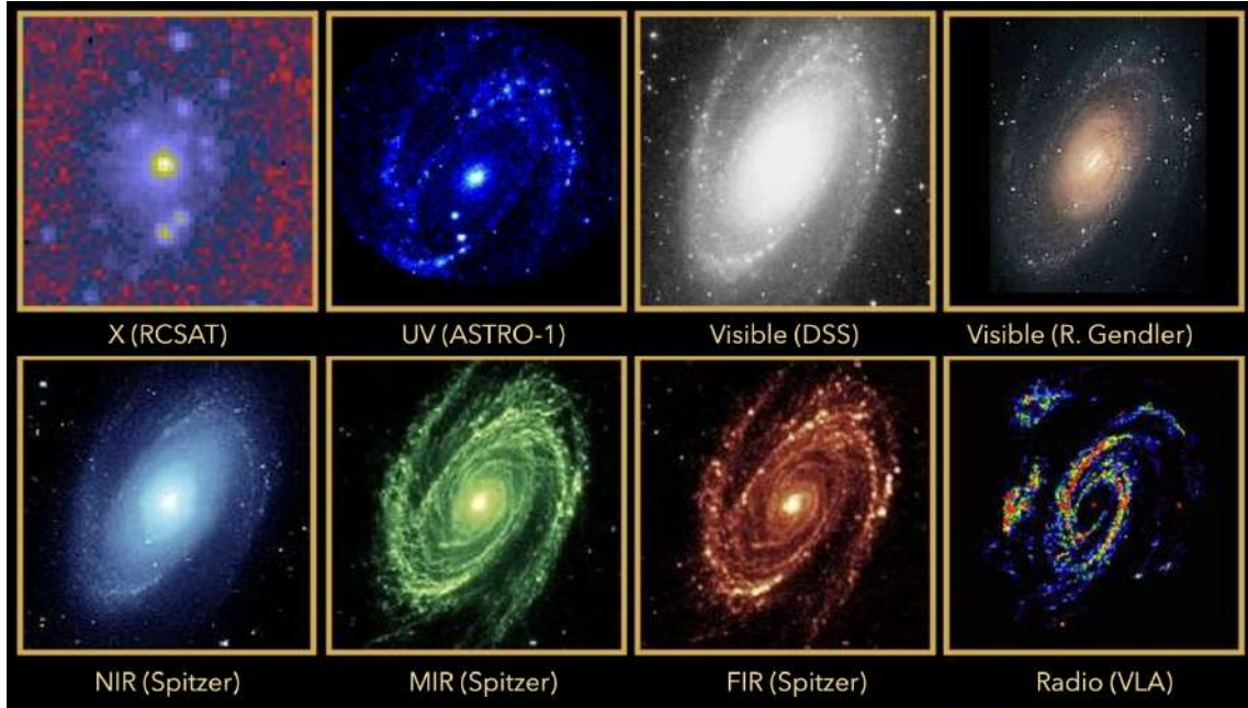
FIGURE 13.4 – La galaxie M81 dans différents domaines du spectre électromagnétique.
