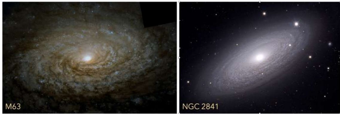
FIGURE 13.7 – Deux exemples de galaxies spirales cotonneuses. M63 à gauche ( HST ) et NGC 2841 à droite ( J.-C. Cuillandre, CFHT ).
