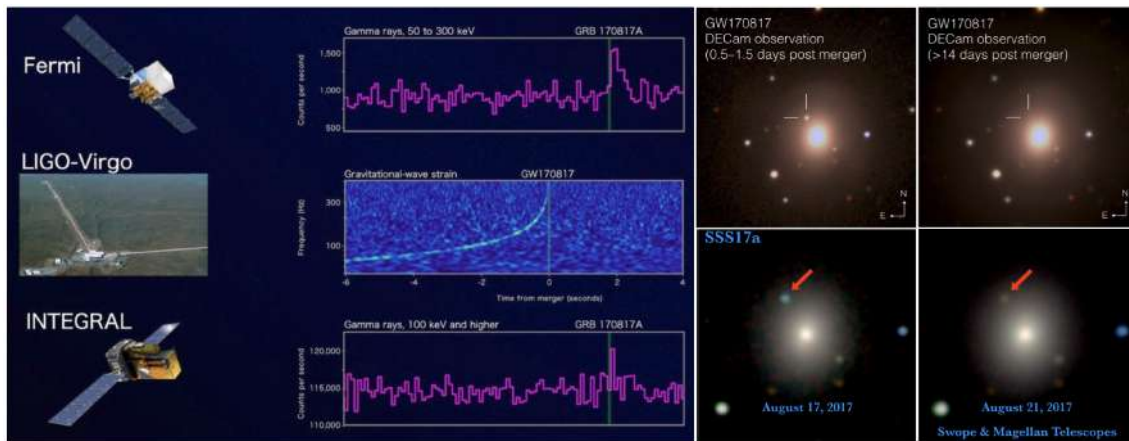
FIGURE 6.1 – Évènement de coalescence de deux étoiles à neutrons . La figure de gauche montre les détections d'ondes gravitationnelles associées à l'évènement détectées avec LIGO-Virgo, les sursauts en rayons \gamma vus par les satellites Fermi et INTEGRAL (Crédit : NASA / GSFC / Caltech / MIT / LIGO / ESA). Les images de droite montrent la position de la source et soulignent sa variation de brillance à différents instants, en optique et en infrarouge proche (Crédit : Soares-Santos et al. and DES Collaboration / 1M2H / UC Santa Cruz and Carnegie Observatories / R. Foley).
